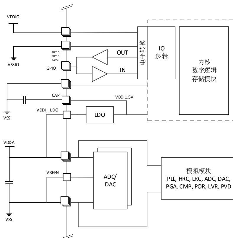
图 3-3 系统电源架构
