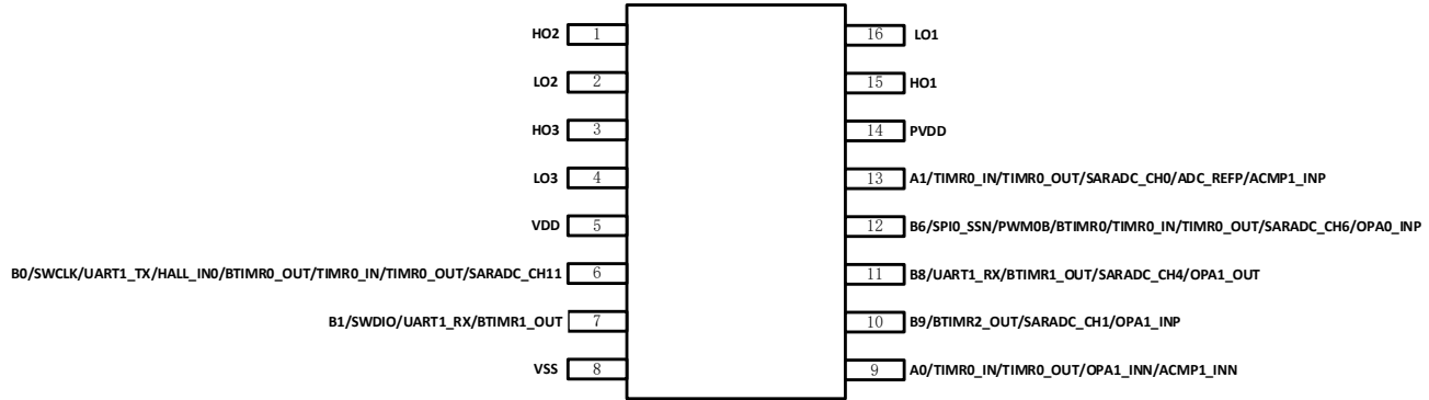
图 5-2 SWM23PQ6M7 封装管脚配置图
