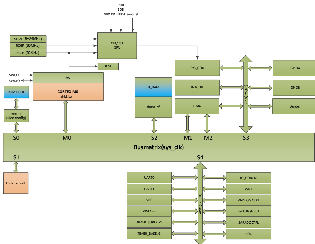
图 3-1 功能方框图
