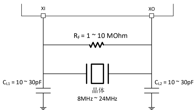
图 9-1 外部晶体振荡器典型电路
