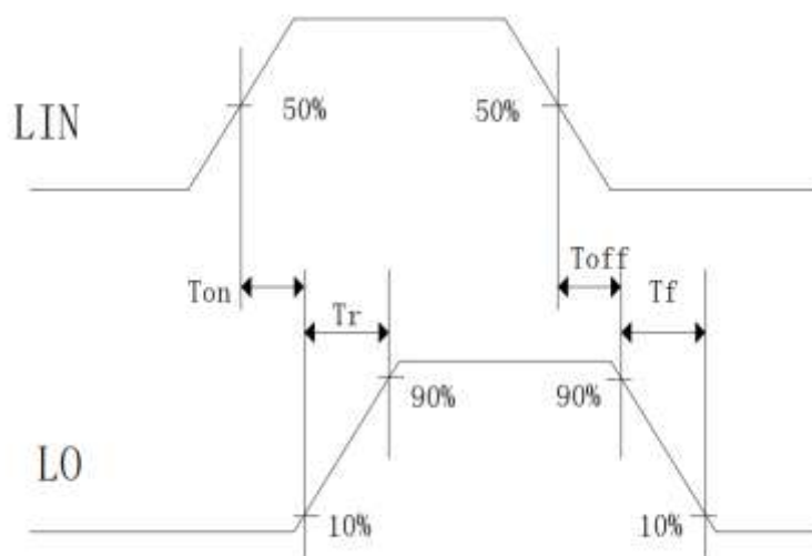
图 9-2 输出 LO 开关时间波形图
