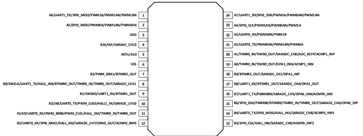
图 5-1 SWM231E6S7 封装管脚配置图
