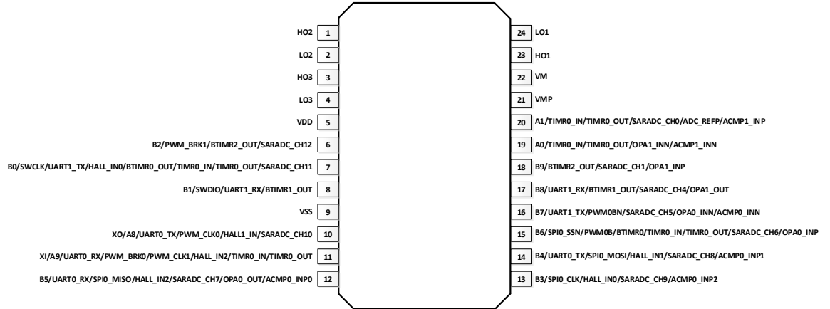
图 5-4 SWM23PE6S7 封装管脚配置图
