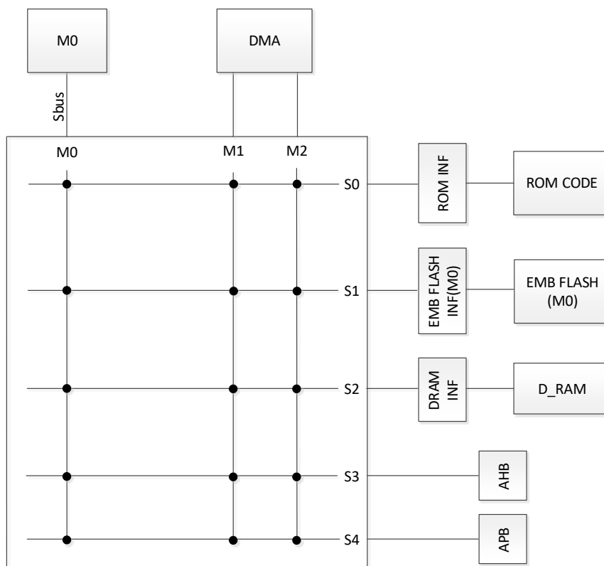
图 3-2 总线矩阵
