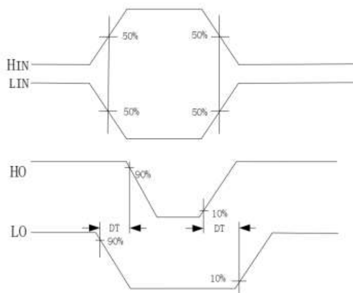
图 9-4 死区时间波形图
