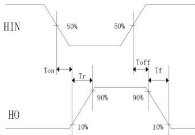
图 9-3 输出 HO 开关时间波形图
