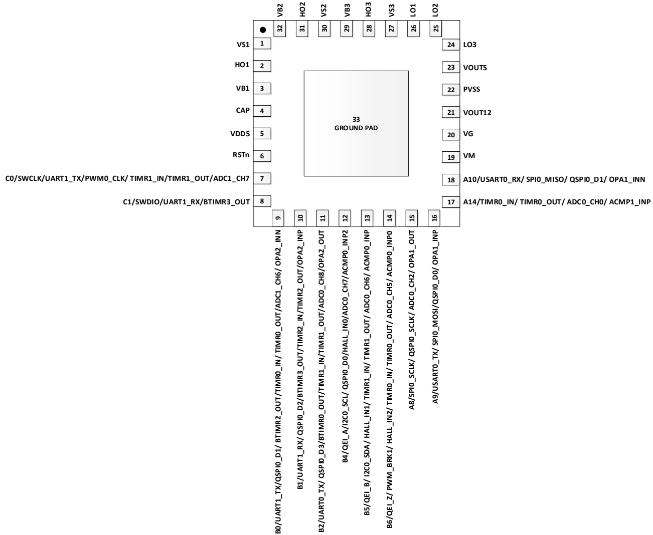
图 5-8 SWM22DK8U7 封装管脚配置图
