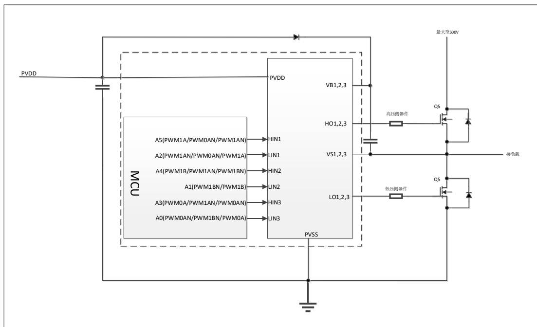
图 8-2 参考应用电路图
