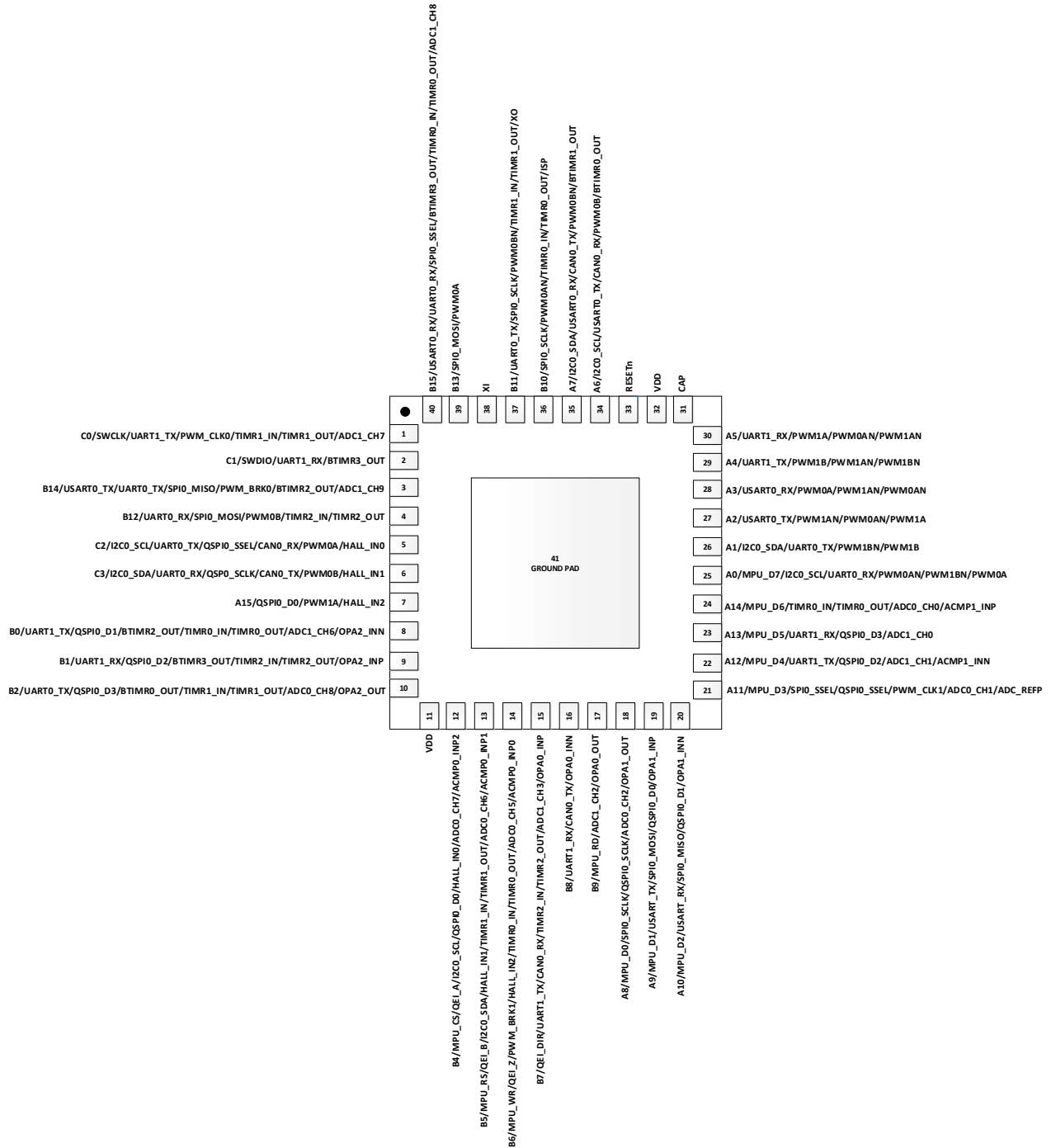
图 5-9 SWM221DBU7 封装管脚配置图 5
