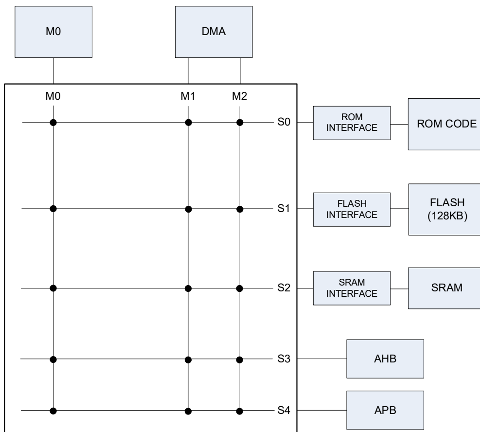
图 4-2 总线矩阵
