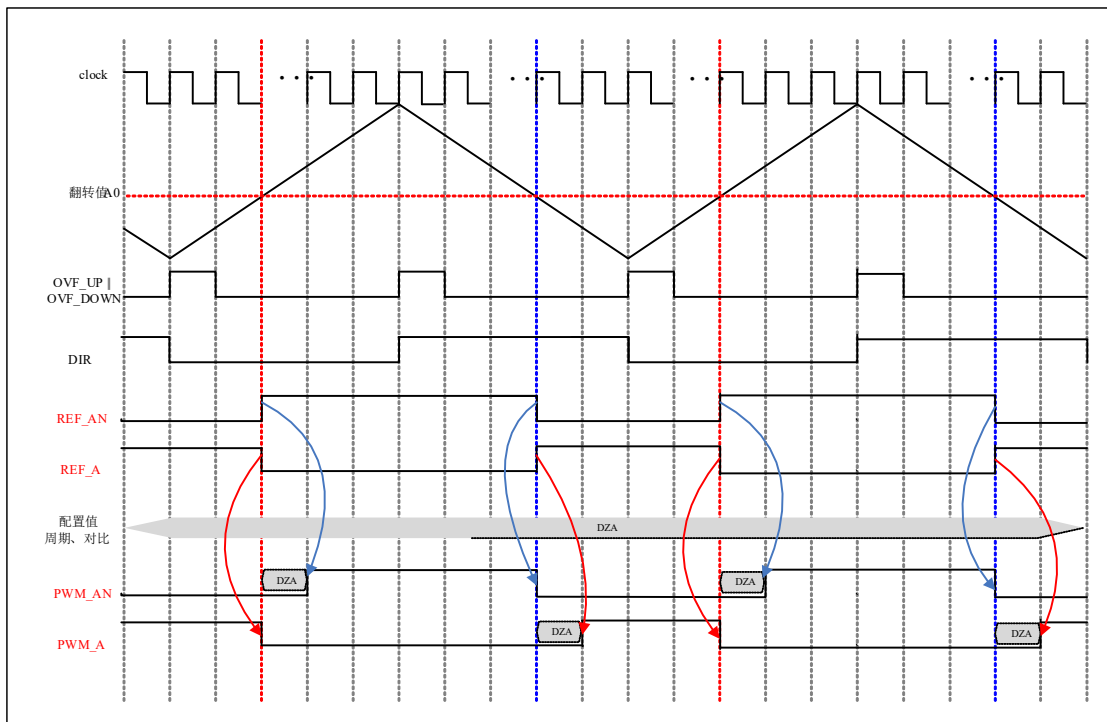
图 6-71 中心对齐模式下 PWM 信号产生波形
