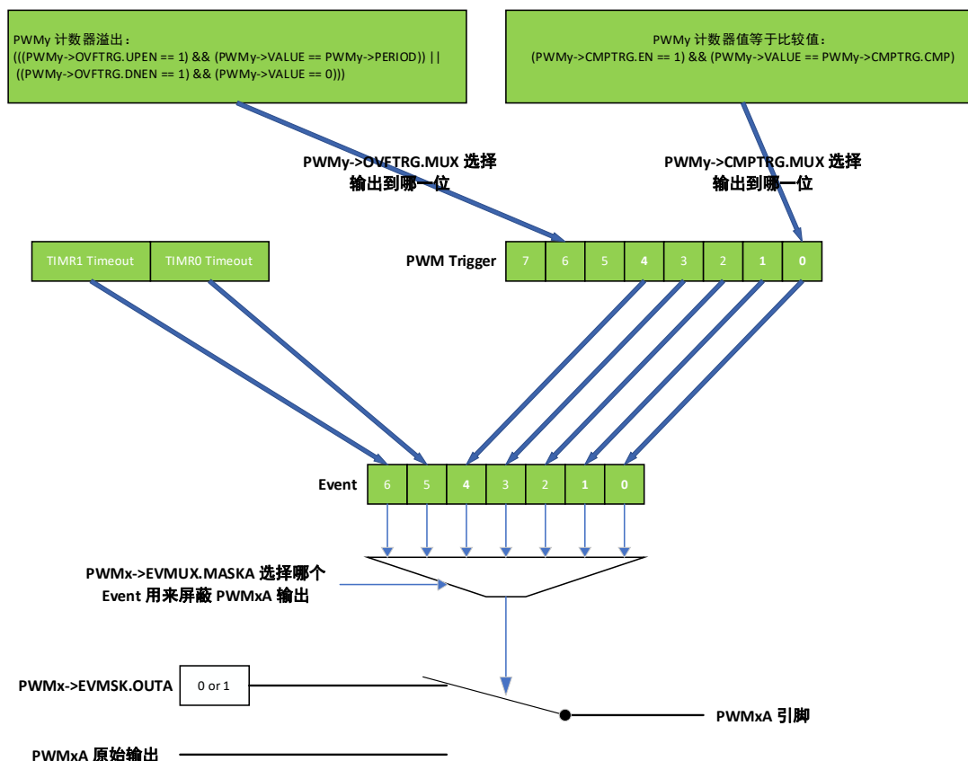
图 6-68 PWM 外部信号配置
