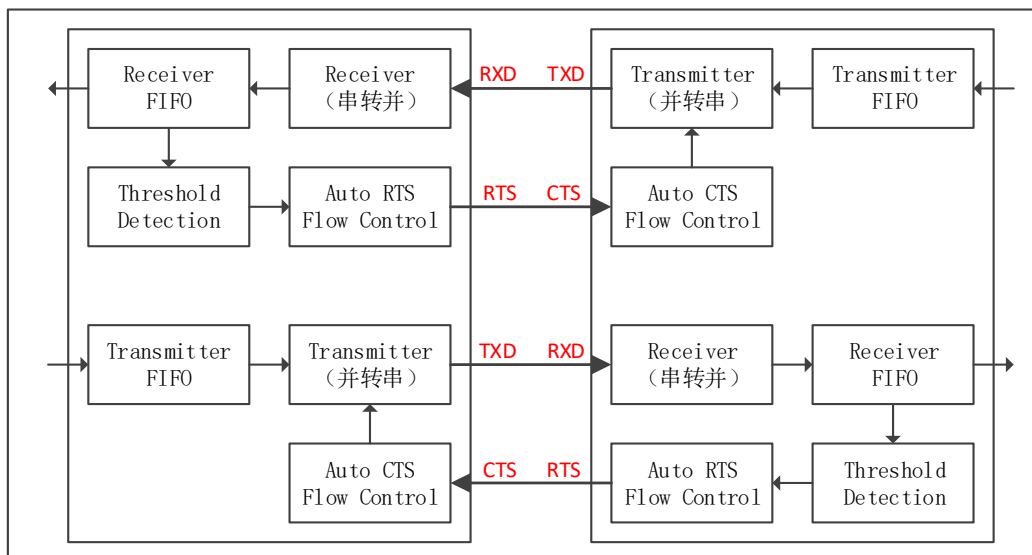
图 6-39 硬件流控
