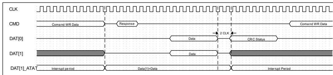
图 6-109 SDIO 写周期时序图
