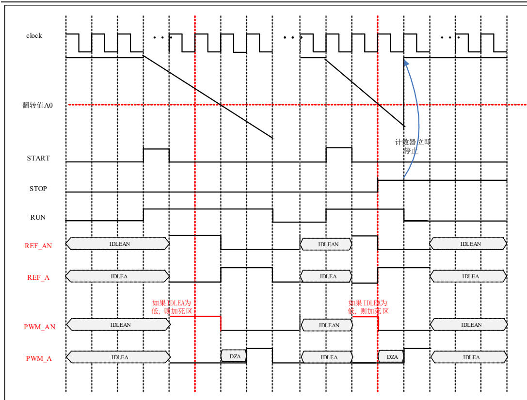
图 6-62 边沿对齐模式下向下计数时计数器启动与停止波形
