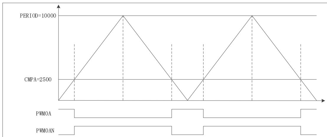
图 6-78 挖坑前波形
