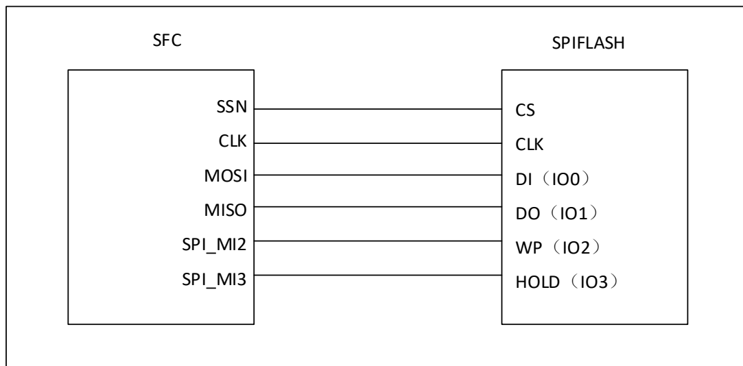
图 6-126 Serial Flash Controller 四线模式外部连接图
