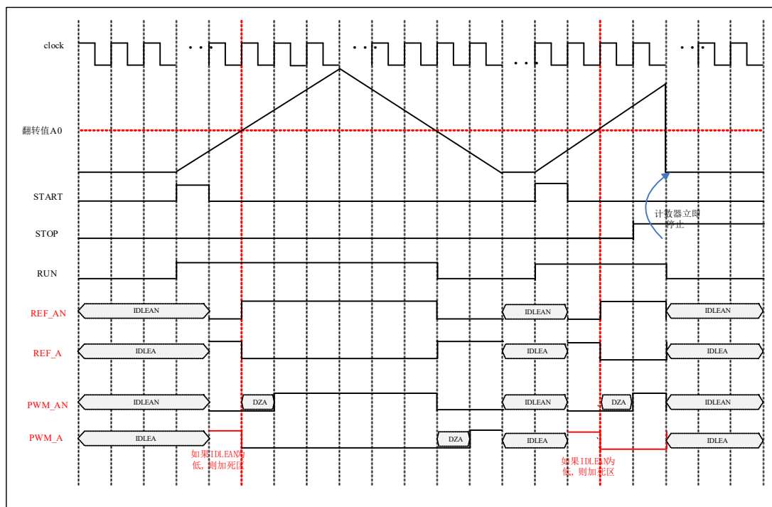
图 6-63 中心对齐模式下计数器启动与停止波形
