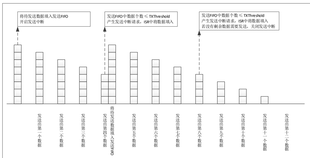
图 6-42 发送 FIFO 示意图
