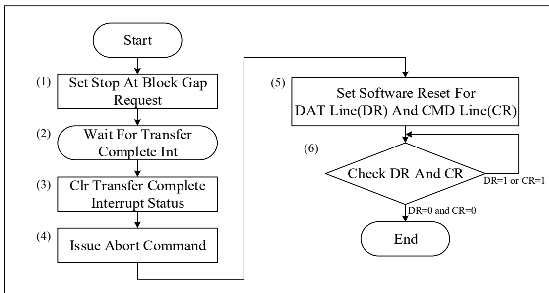
图 6-108 SDIO 同步中止传输示意图
