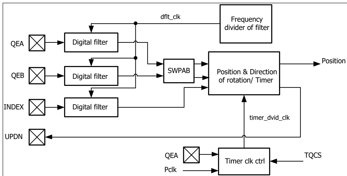
图 6-19 QEI 模块结构框图
