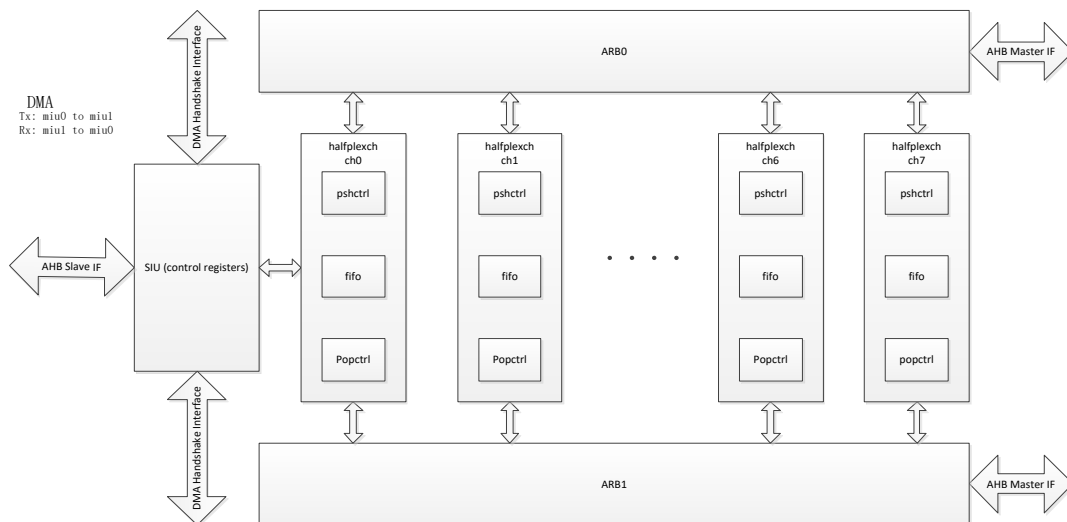
图 6-87 DMA 模块结构图
