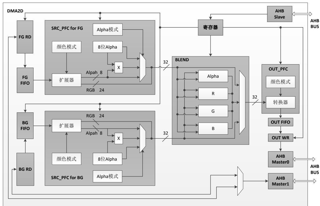
图 6-99 DMA2D 模块结构框图
