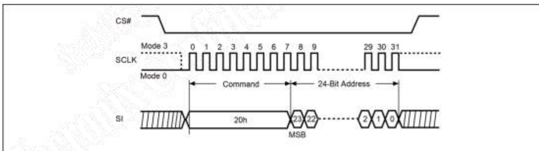
图 6-122 Sector 擦时序图
