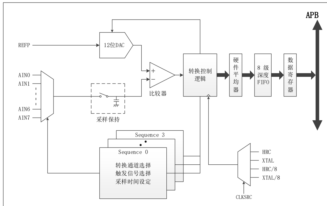
图 6-80 ADC 模块结构框图
