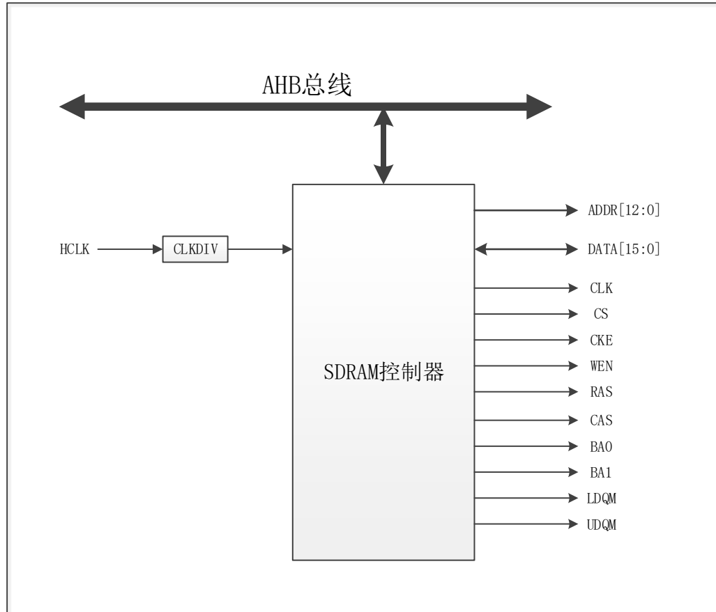
图 6-101 SDRAMC 模块结构框图
