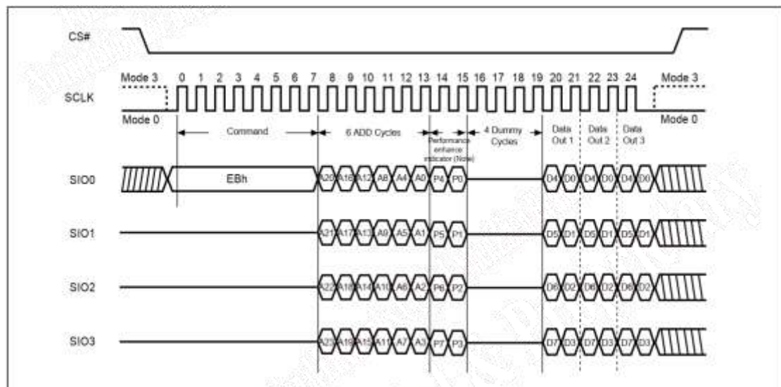
图 6-119 四线 IO 读模式时序图
