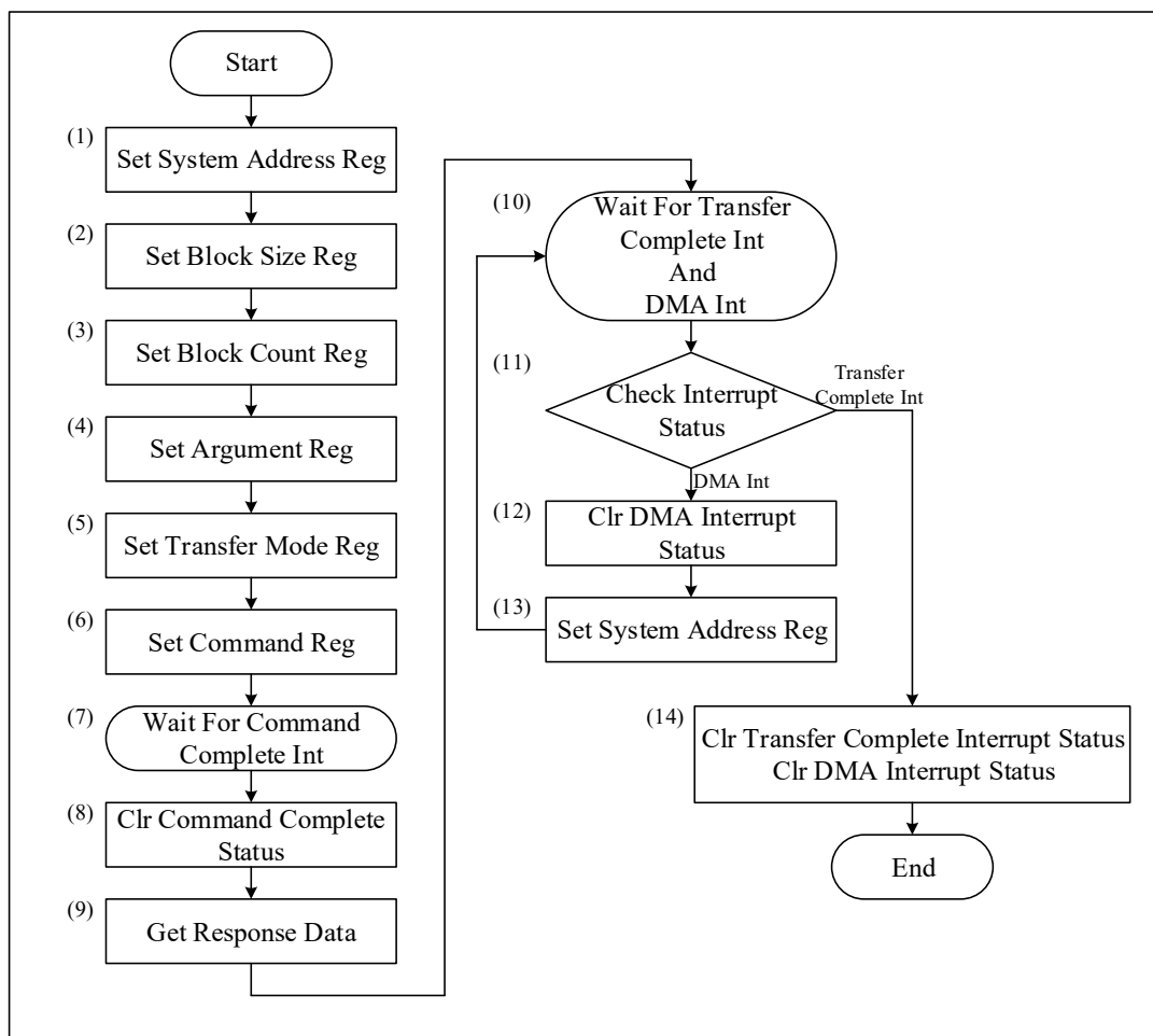
图 6-106 SDIO 使用 DMA 传输示意图
