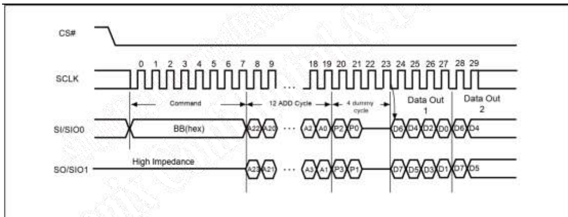
图 6-118 2xIO 读模式时序图
