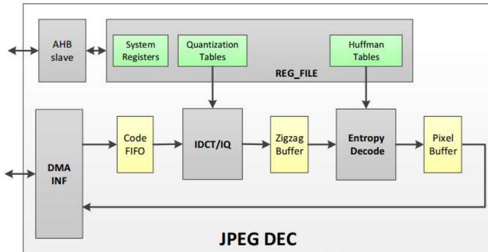
图 6-98 JPEG 模块结构示意图
