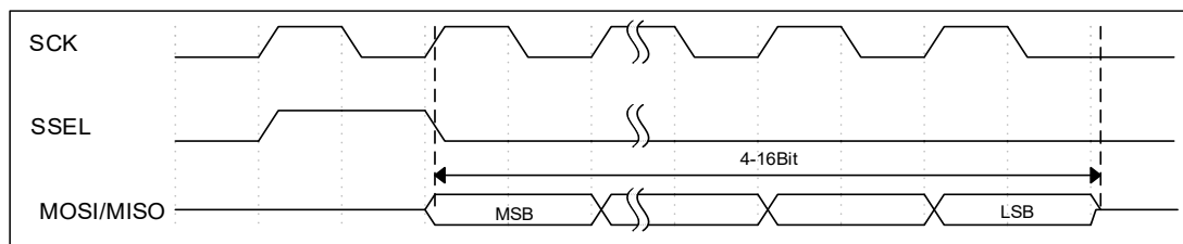
图 6-50 SSI 模式单次输出波
