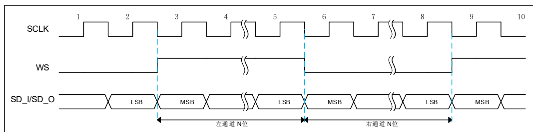
图 6-58 PCM 长帧数据格式时序图 (PCMSYNW = 1)
