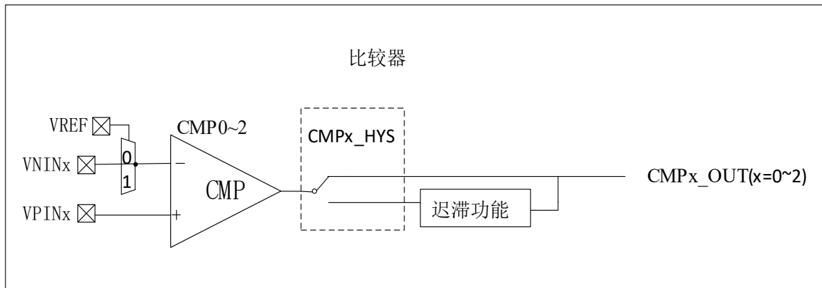
图 6-128 比较器框图
