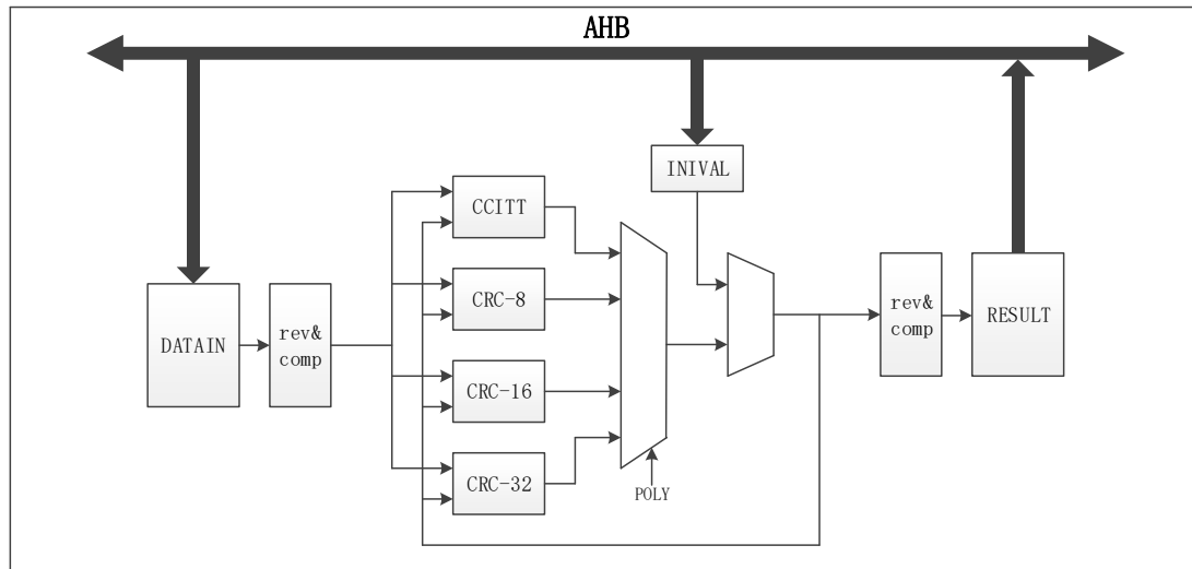
图 6-91 CRC 结构框图
