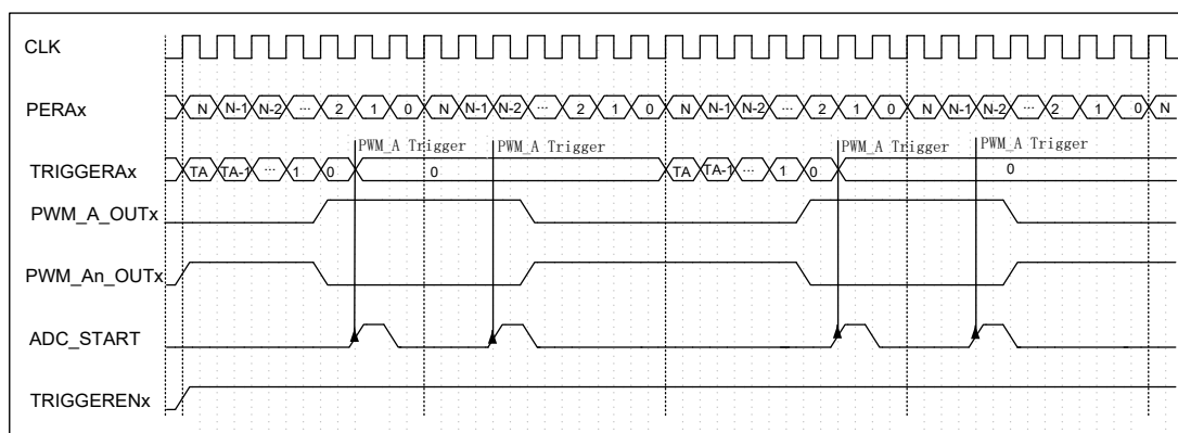
图 6-83 A 和 An 中心对称互补模式下 PWM 触发 ADC 采样示意图
