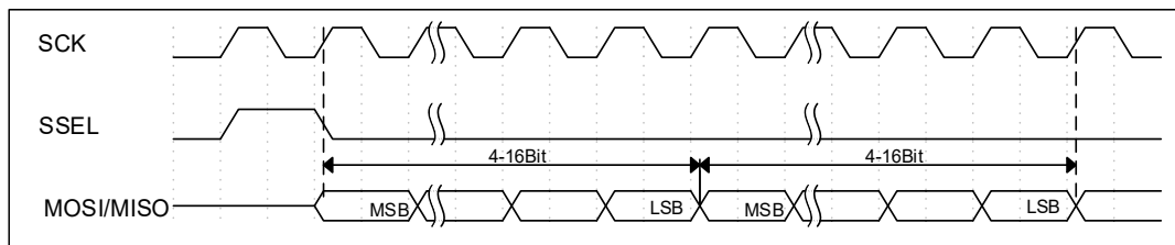
图 6-51 SSI 模式连续输出波形
