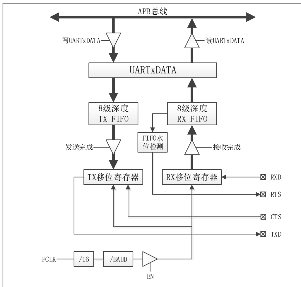
图 6-32 UART 模块结构图
