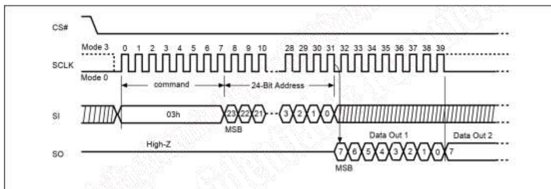
图 6-117 标准读模式时序图
