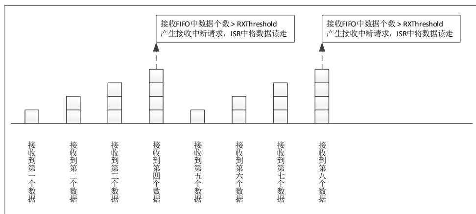
图 6-40 对方发送 8 个数据接收 FIFO 示意图
