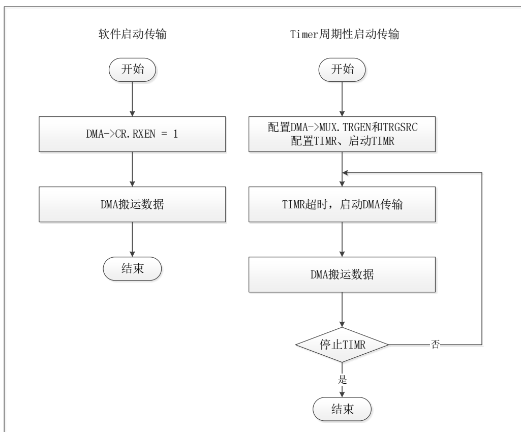
图 6-90 DMA 启动方式
