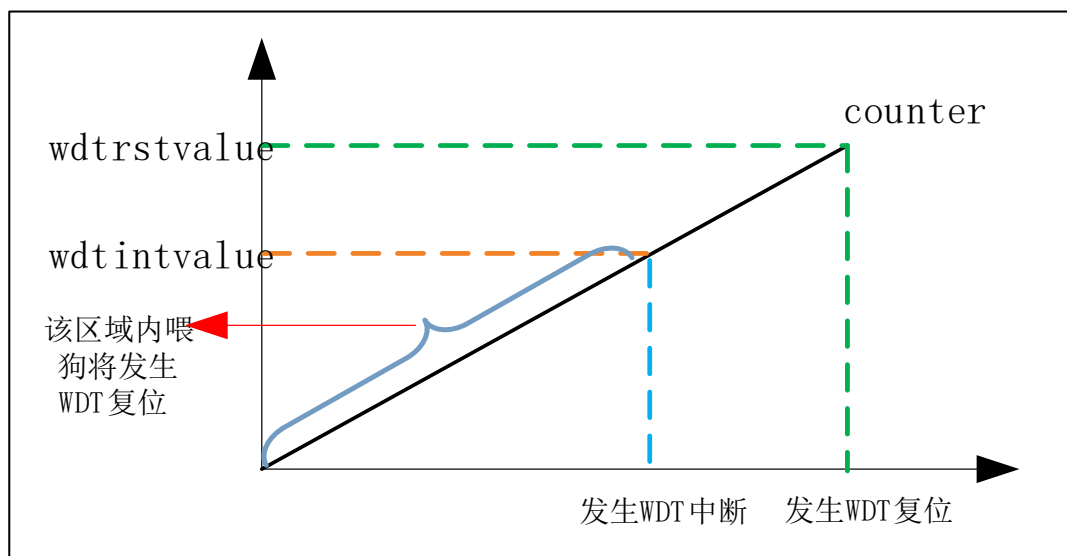
图 6-27 门狗发生中断及复位与计数值之间的关系示意图
