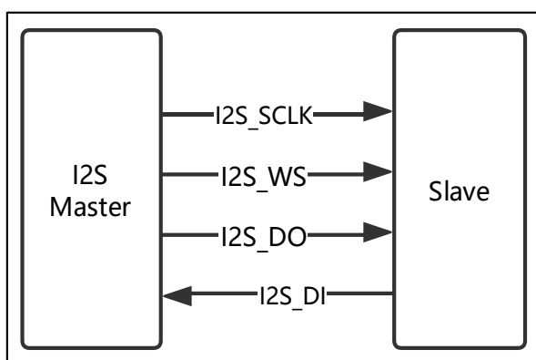
图 6-52 主机模式接口框图
