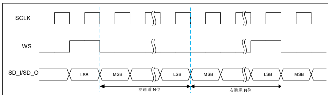
图 6-56 PCM 短帧数据格式时序图
