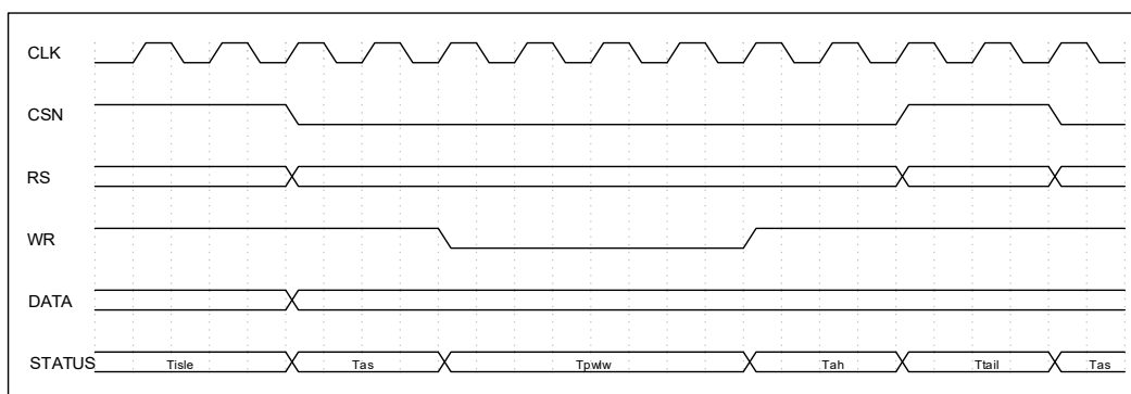
图 6-94 LCDC 模块 MPU 接口时序图
