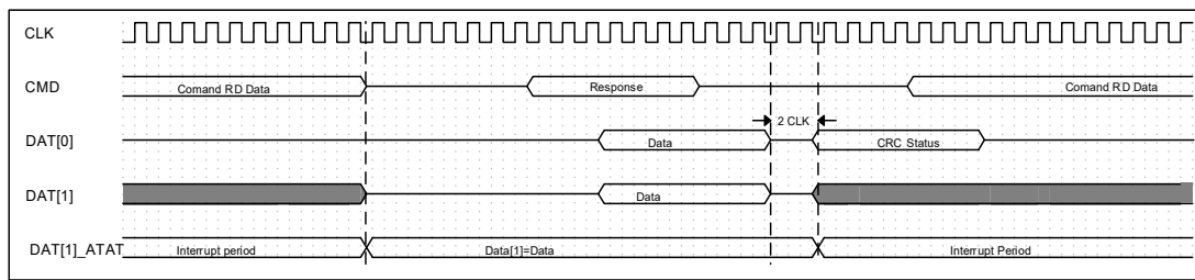
图 6-110 SDIO 读周期时序图
