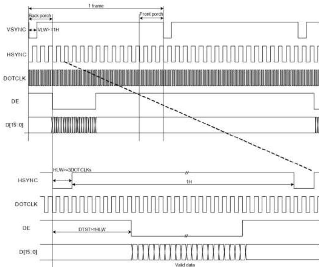
图 6-96 16bit RGB 接口模式时序图
