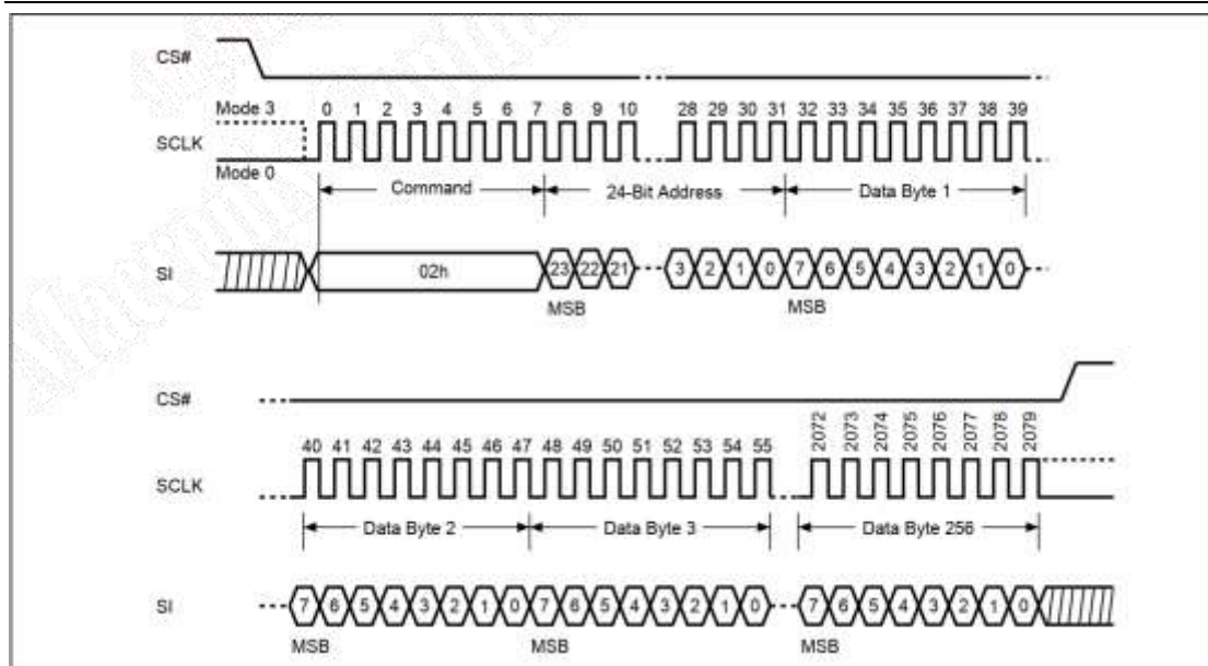
图 6-120 标准写(page)模式时序图
