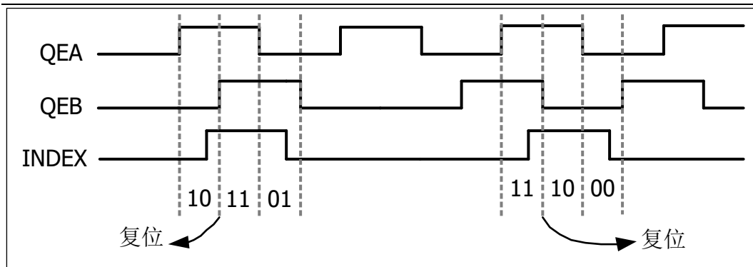
图 6-24 QEI 计数器索引复位模式
