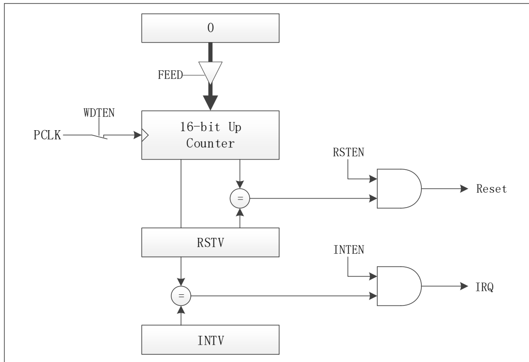
图 6-26 WDT 模块结构框图
