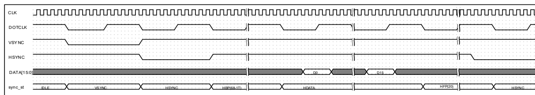
图 6-95 LCD 模块 SYNC 接口时序图
