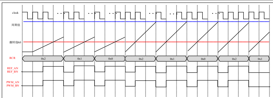
图 6-75 重复计数功能波形图
