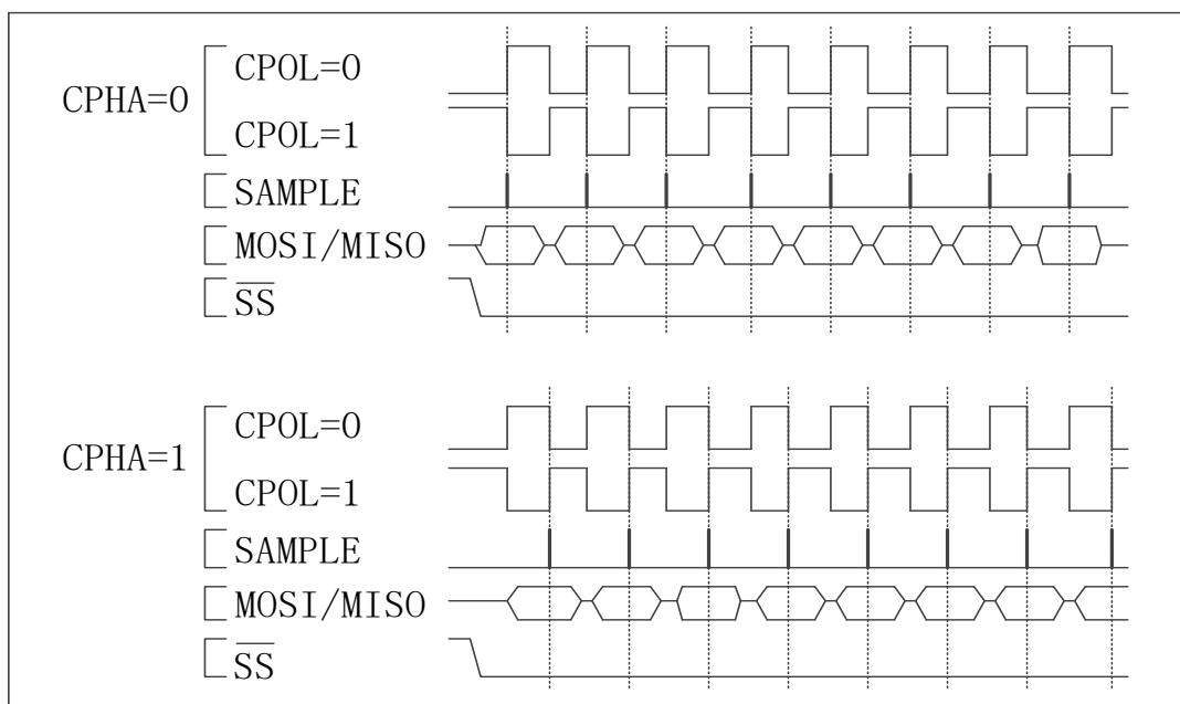
图 6-49 SPI 模式波形图
