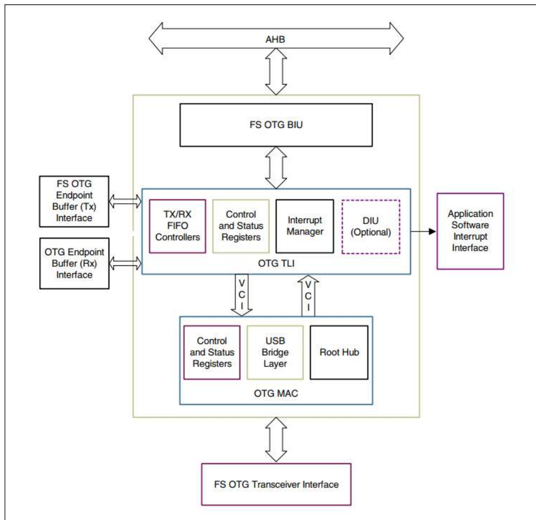
图 6-113 USB 框图
