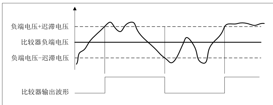
图 6-129 比较器迟滞功能示意图
