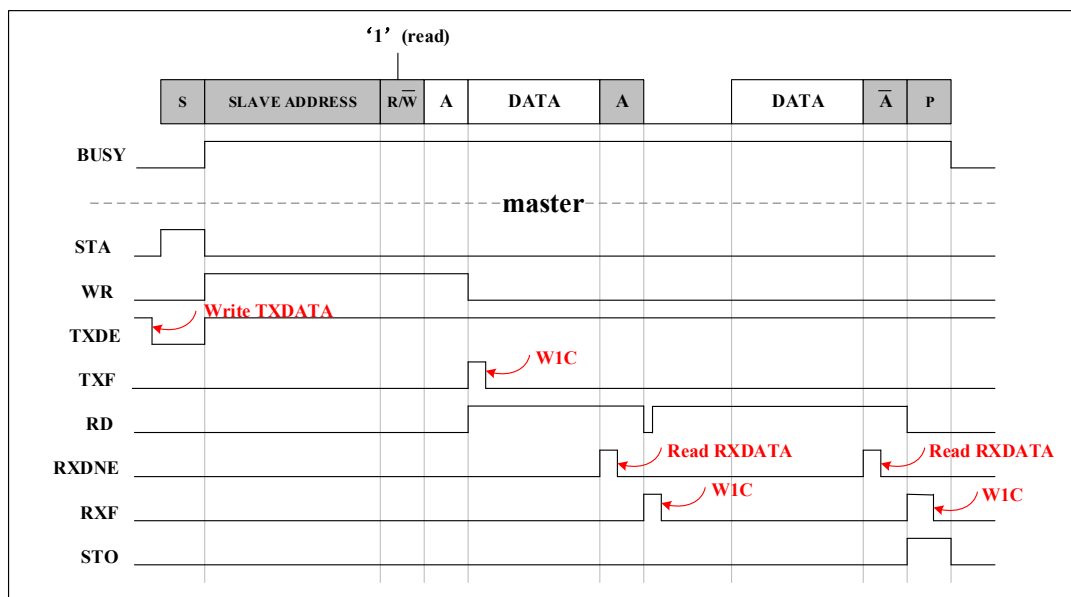
图 6-46 Master 寄存器时序示意图
