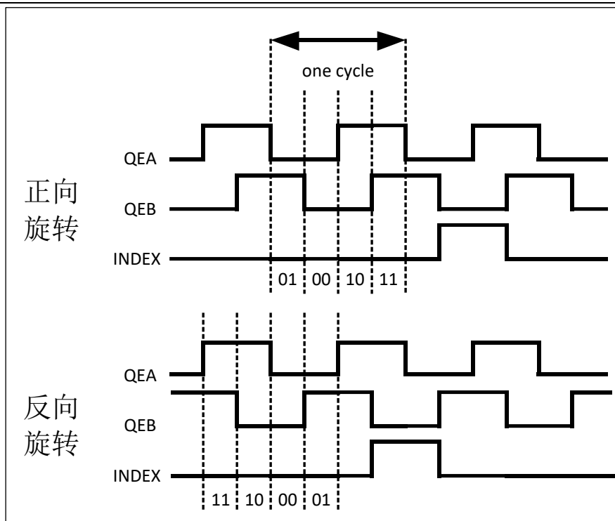
图 6-21 三相信号正向/反向旋转时序关系
