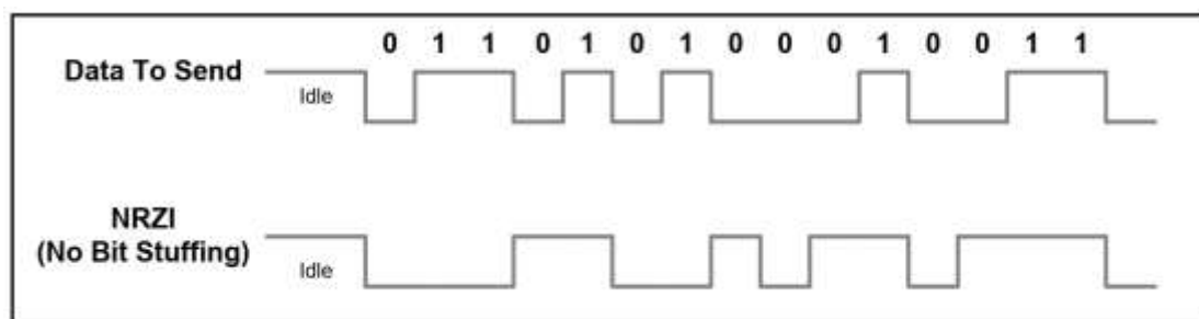
图 6-114 NRZI 编码的逻辑电平
