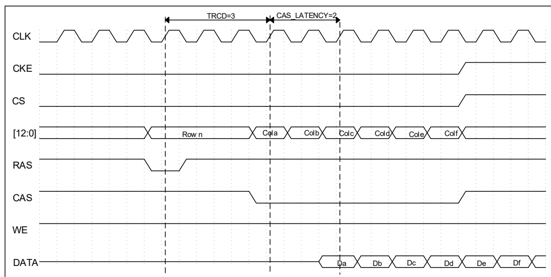
图 6-104 SDRAMC 读访问周期示意图
