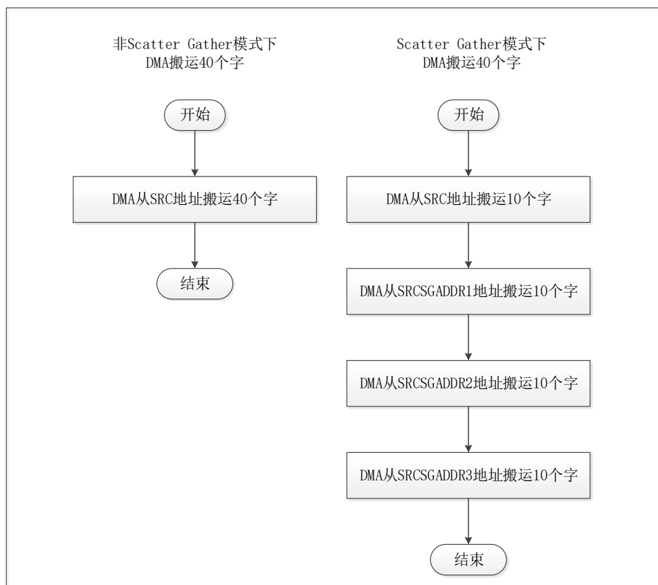
图 6-88 DMA 搬运 40 个字流程图
