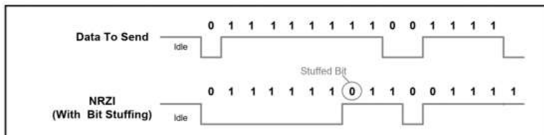
图 6-115 带位填充的 NRZI 编码的逻辑电平
