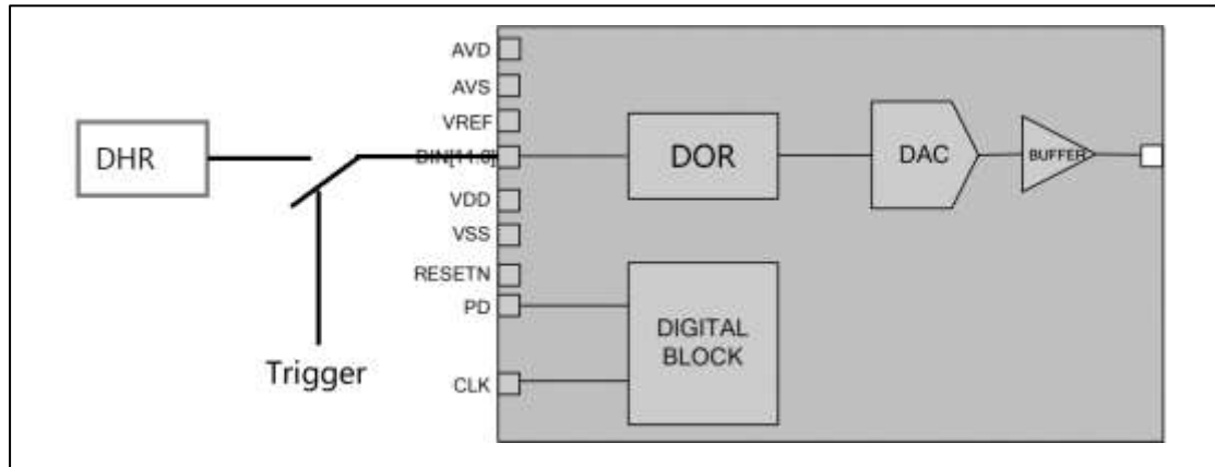
图 6-112 DAC 模块结构框图
