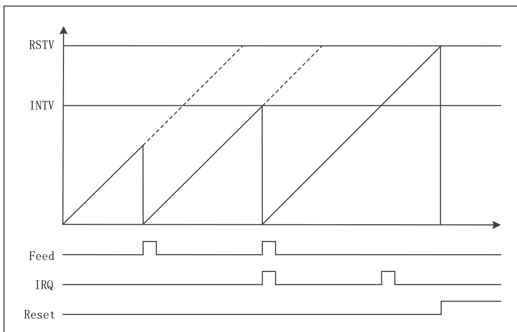
图 6-28 WDT 工作示意图
