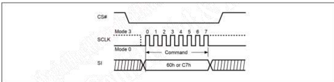
图 6-125 Chip 擦操作时序图
