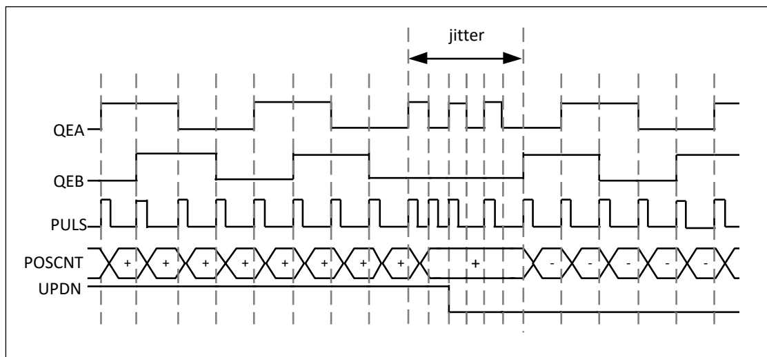
图 6-22 正交编码器 x4 计数模式示意图
