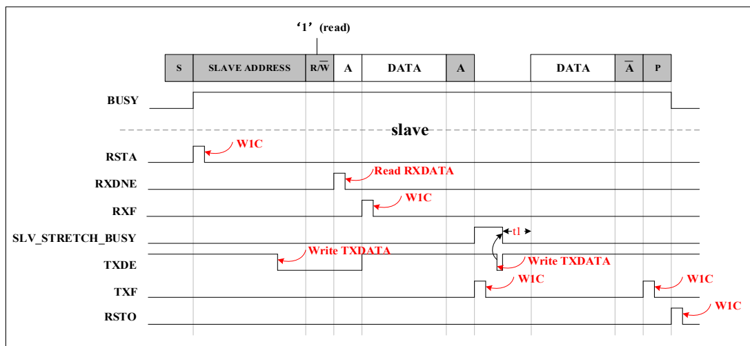
图 6-47 Slave 寄存器时序示意图
