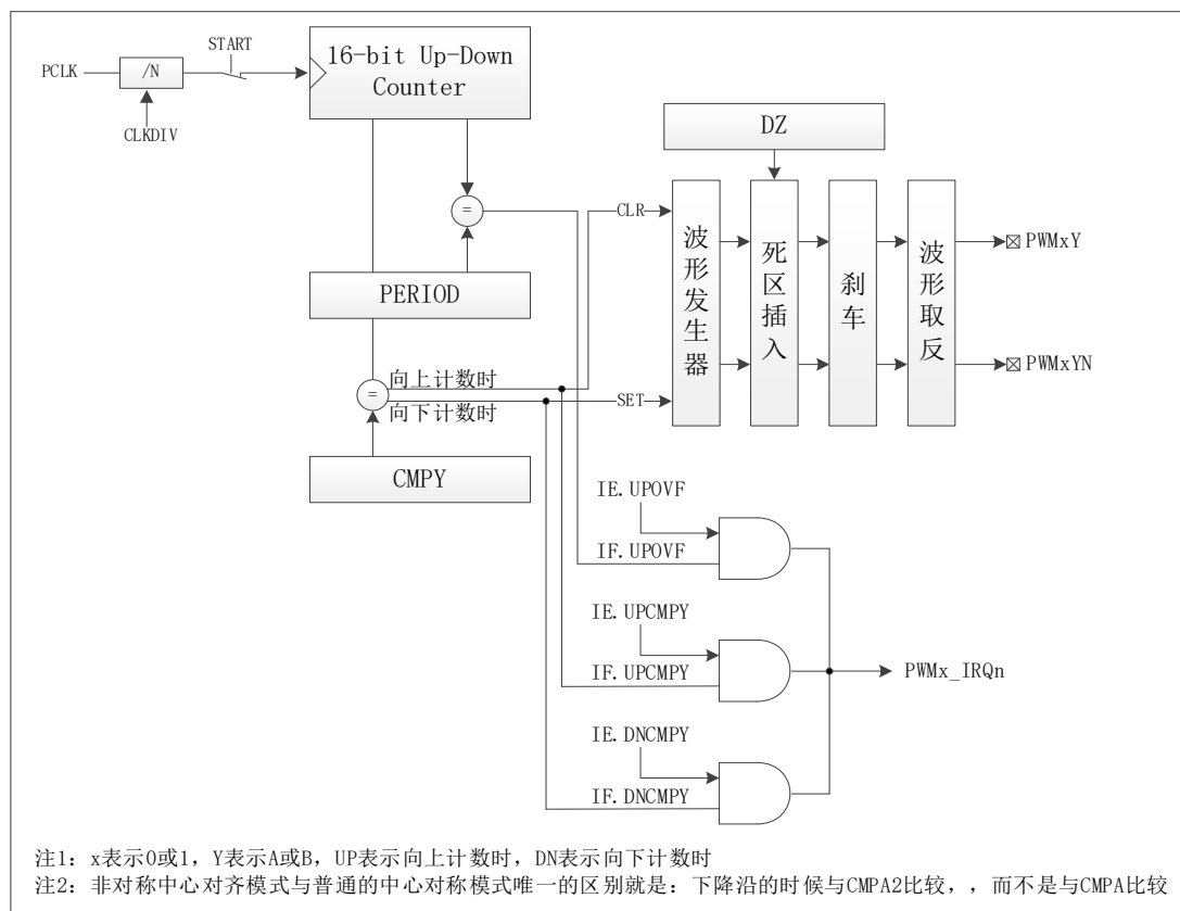
图 6-59 PWM 模块结构框图
