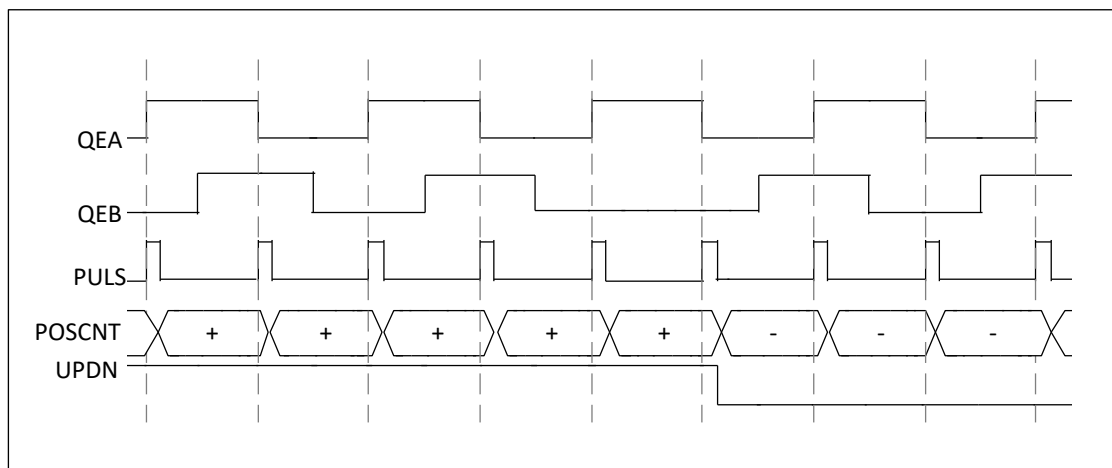
图 6-23 正交编码器 x2 计数模式示意图
