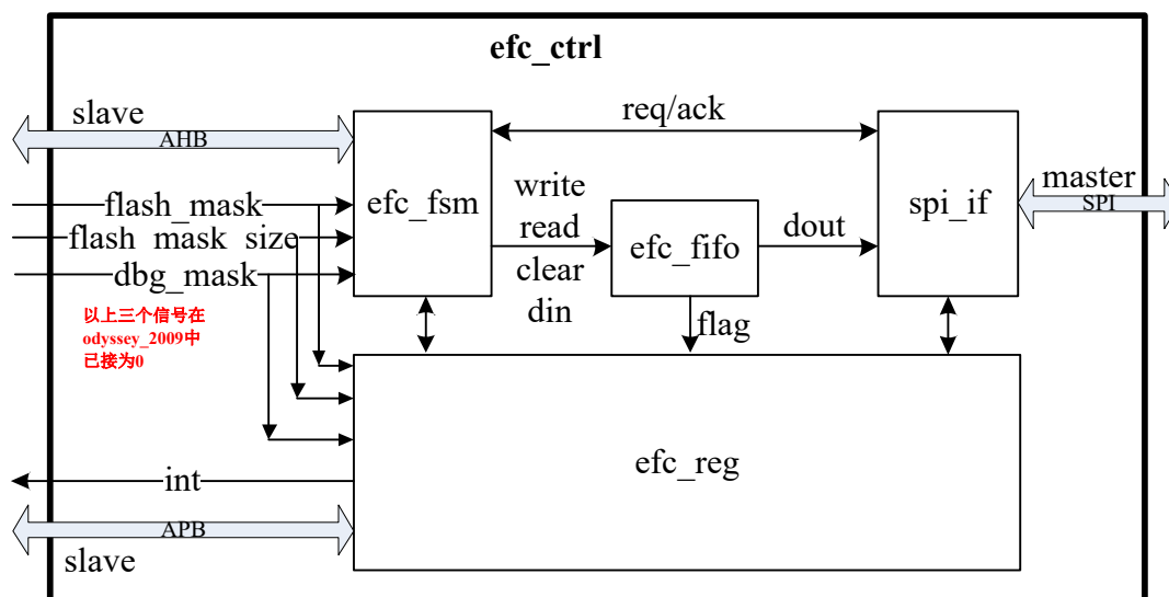
图 6-116 模块结构框图
