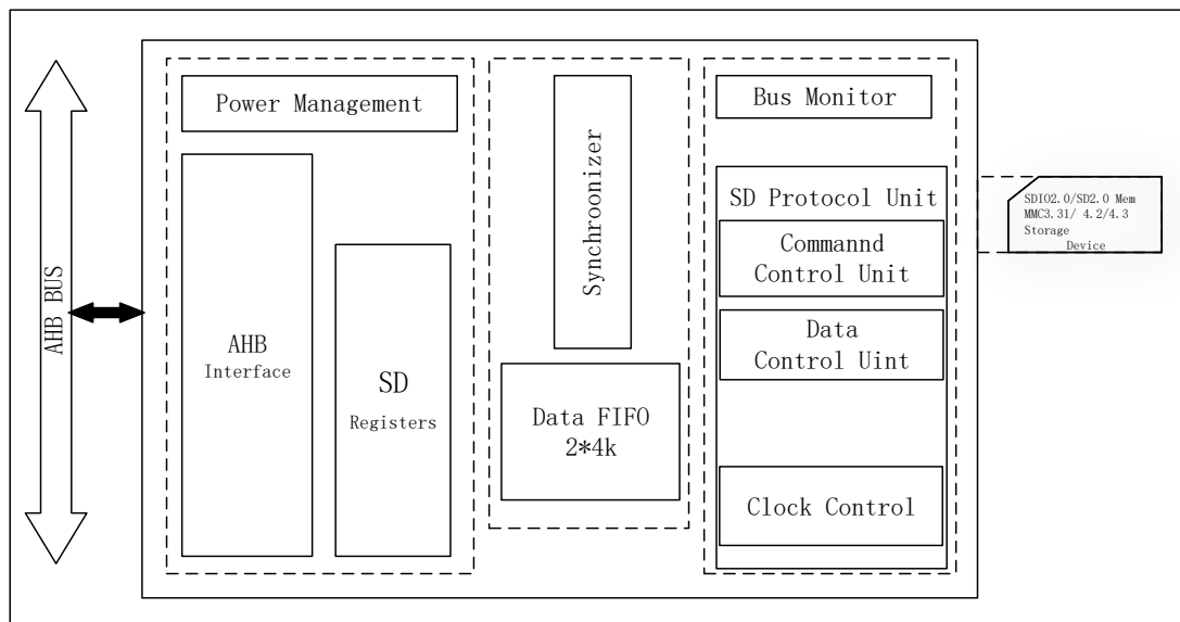
图 6-105 SDIO 模块结构框图
