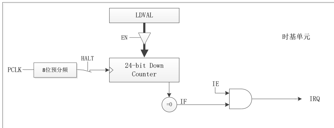
图 6-15 BTIMER 模块结构框图
