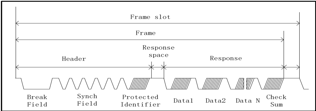
图 6-35 LIN Fram 示意图
