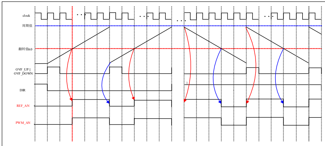
图 6-70 边沿对齐模式下 PWM 信号产生波形
