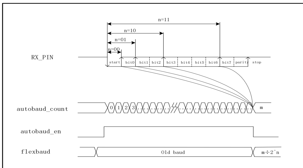
图 6-34 自动波特率示意图
