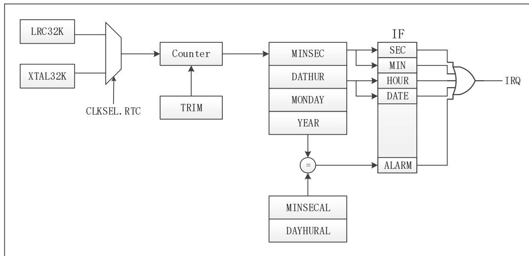
图 6-31 RTC 模块结构框图
