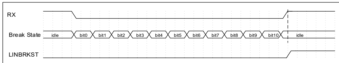
图 6-38 Break 信号足够长示意图
