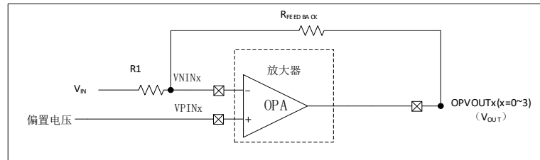
图 6-131 放大器框图
