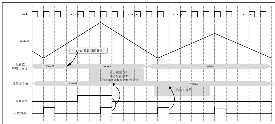
图 6-69 计数器重载波形
