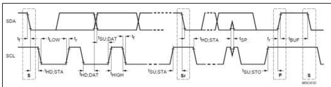
图 6-45 Master SCL 周期配置示意图
