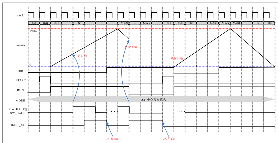
图 6-67 硬件刹车控制和软件刹车控制计数器计数情况
