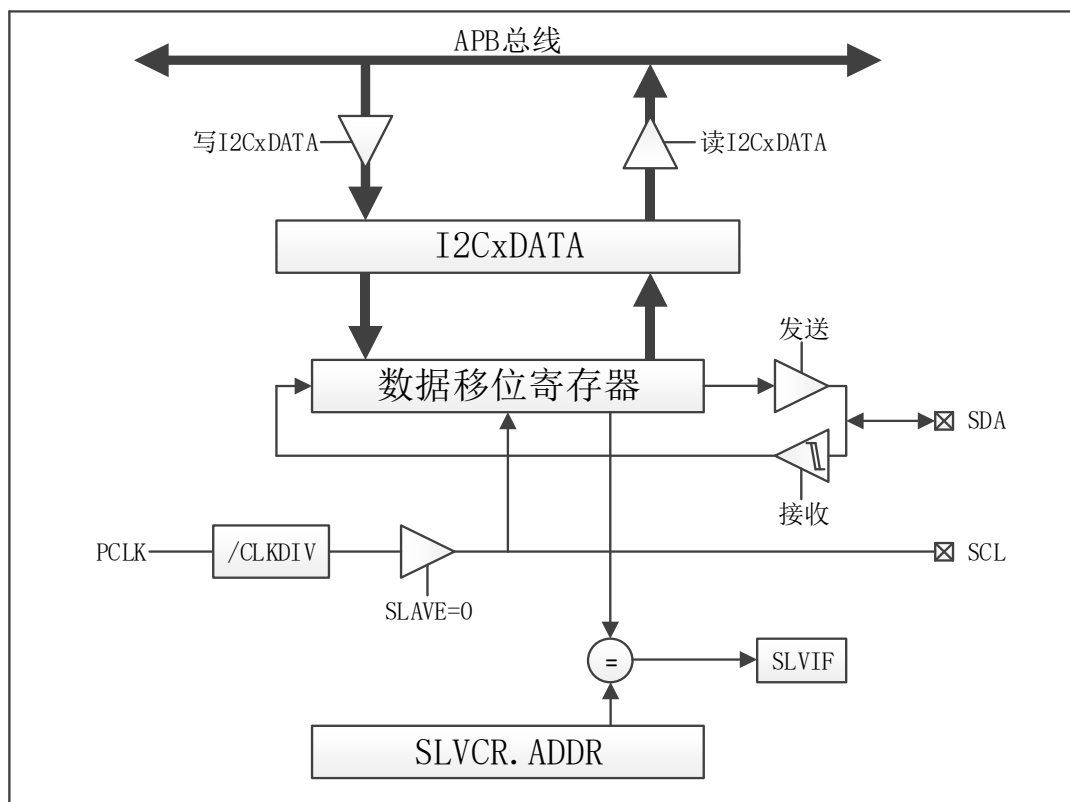
图 6-43 I2C 模块结构框图
