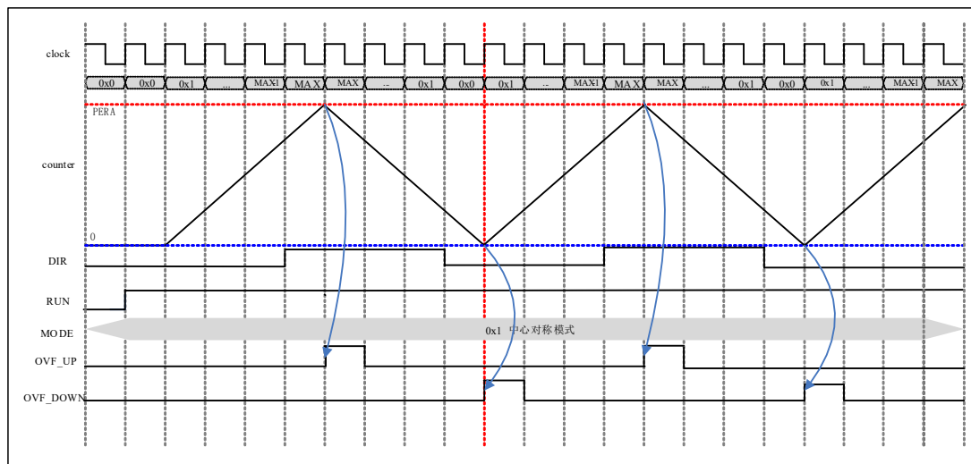
图 6-66 中心对称模式下计数器计数过程波形
