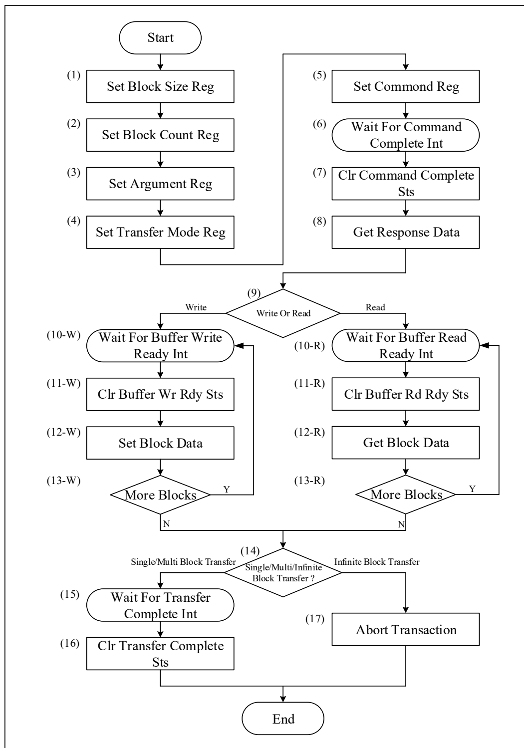
图 6-107 SDIO 不使用 DMA 传输示意图
