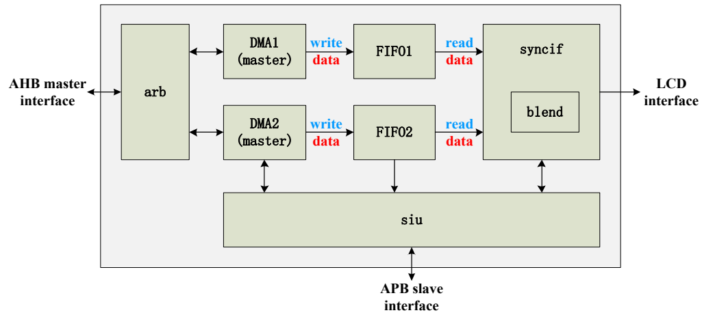
图 6-93 LCDC 模块结构示意图
