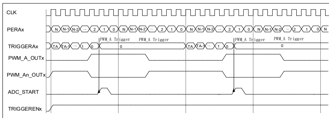
图 6-76 PWM 触发 ADC 采样示意图
