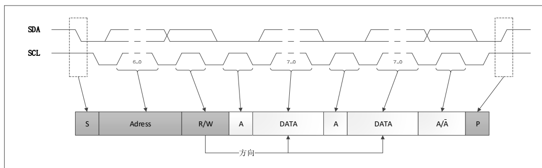
图 6-44 I2C 通信示意图
