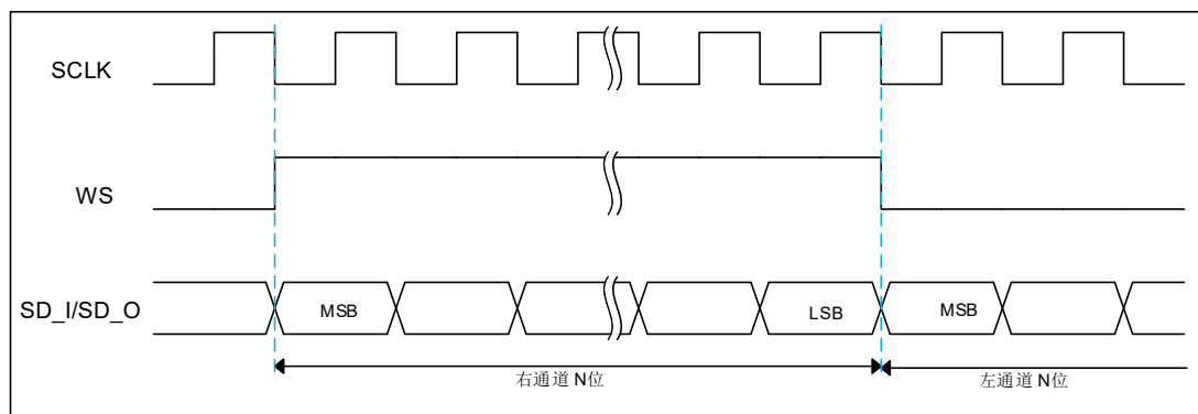
图 6-55 MSB 对齐数据格式时序图
