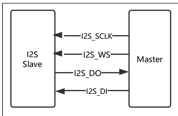
图 6-53 从机模式接口框图
