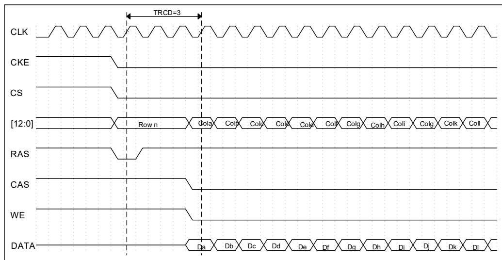
图 6-103 SDRAMC 写访问周期示意图
