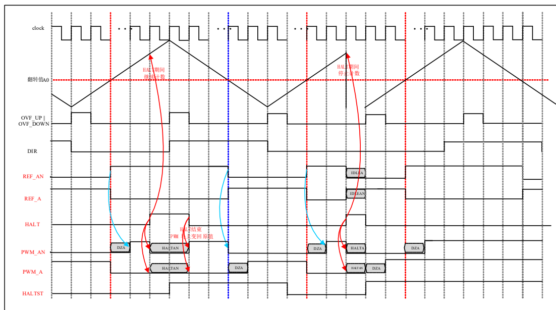
图 6-73 BRK 中心对齐模式下 PWM 信号产生波形
