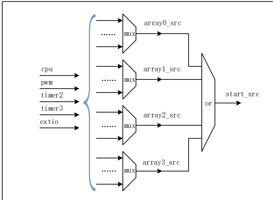
图 6-82 ADC 触发源选择示意图
