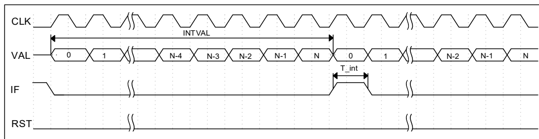
图 6-30 WDT 配置为中断模式波形图
