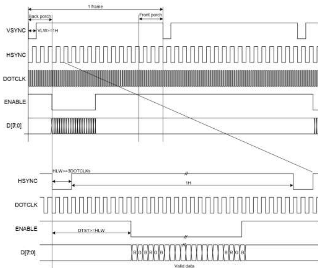
图 6-97 串行同步模式时序图
