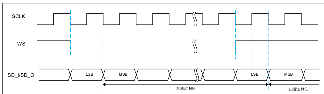
图 6-54 philips 数据格式时序图
