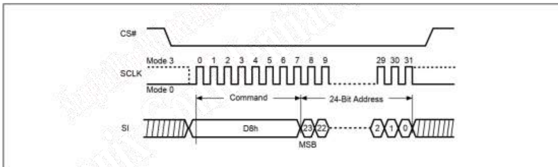
图 6-124 Block(64K)擦操作时序图
