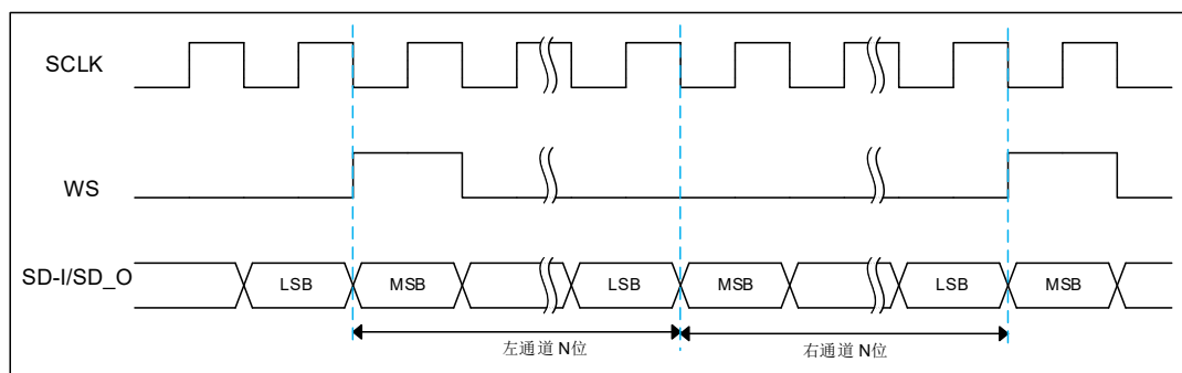
图 6-57 PCM 长帧数据格式时序图 (PCMSYNW = 0)
