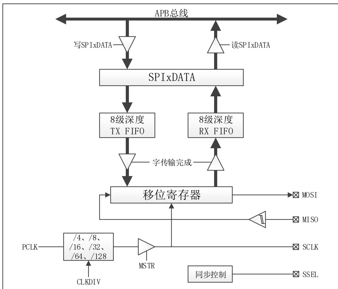
图 6-48 SPI 模块结构框图
