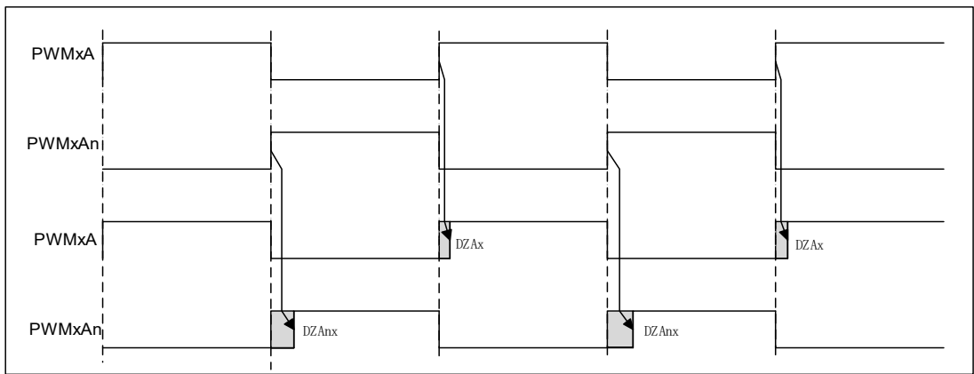
图 6-60 PWM 死区示意图
