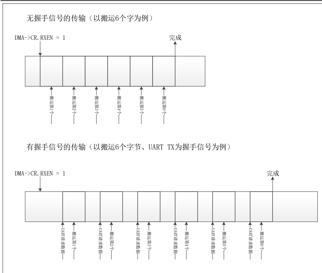
图 6-89 握手、非握手信号传输图
