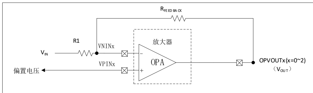
图 6-132 典型放大电路
