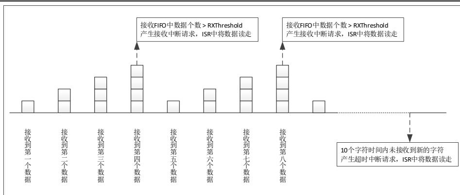
图 6-41 对方发送 9 个数据接收 FIFO 示意图
