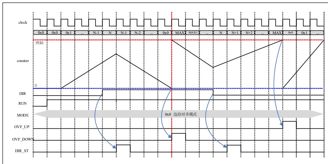
图 6-65 边沿对齐模式下计数器计数过程波形
