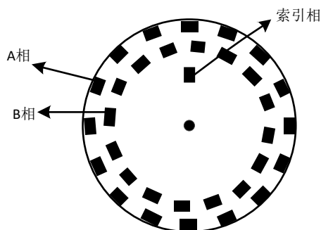
图 6-20 增量式正交编码盘示意图
