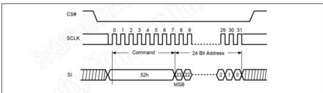
图 6-123 Block(32K)擦操作时序图
