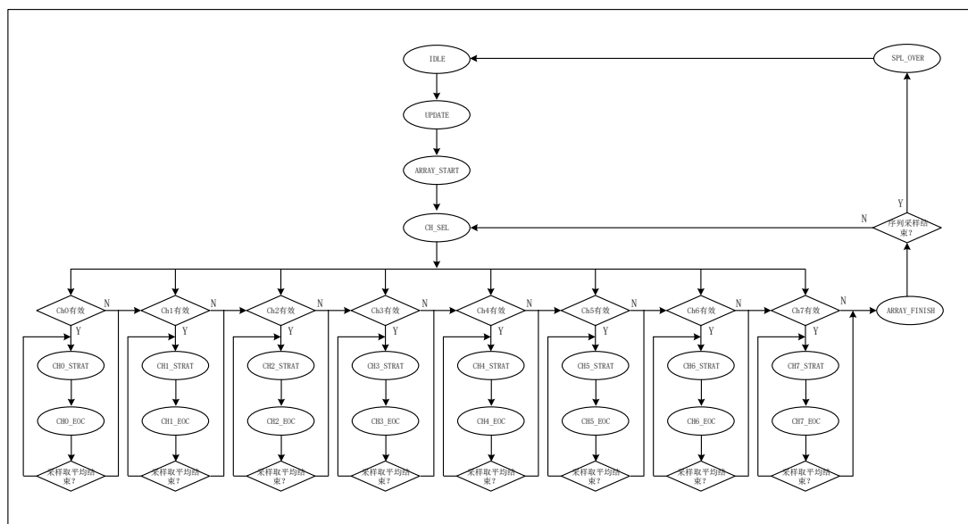
图 6-81 ADC 采样流程图
