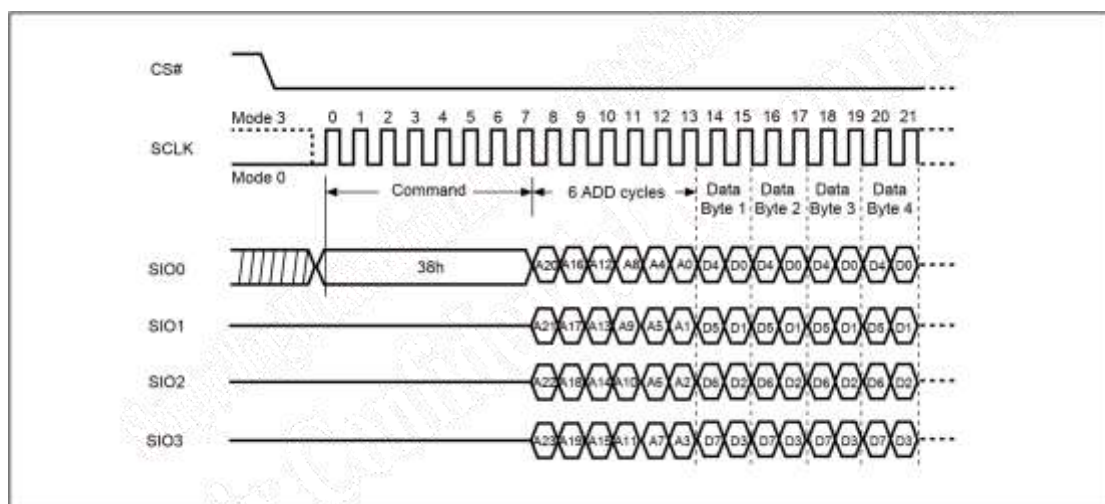
图 6-121 四线 IO 写(page)模式时序图
