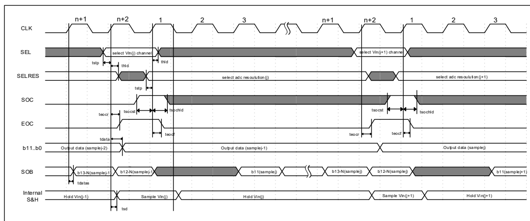
图 6-86 ADC 连续采样示意图
