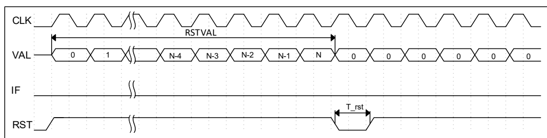
图 6-29 WDT 配置为 RESET 模式波形图
