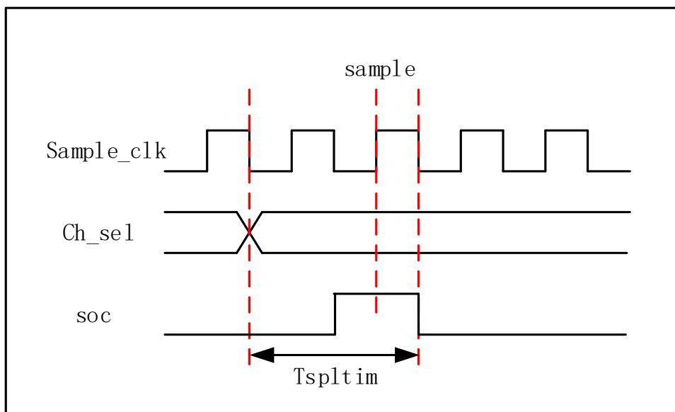
图 6-84 ADC 采样建立时间
