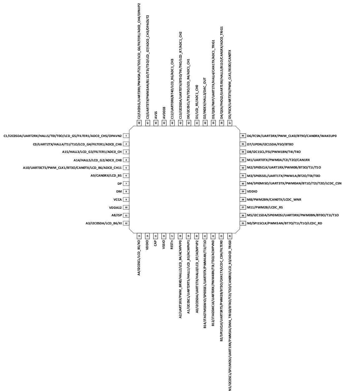
图 5-6 SWM34SCET6 LQFP48 管脚排布
