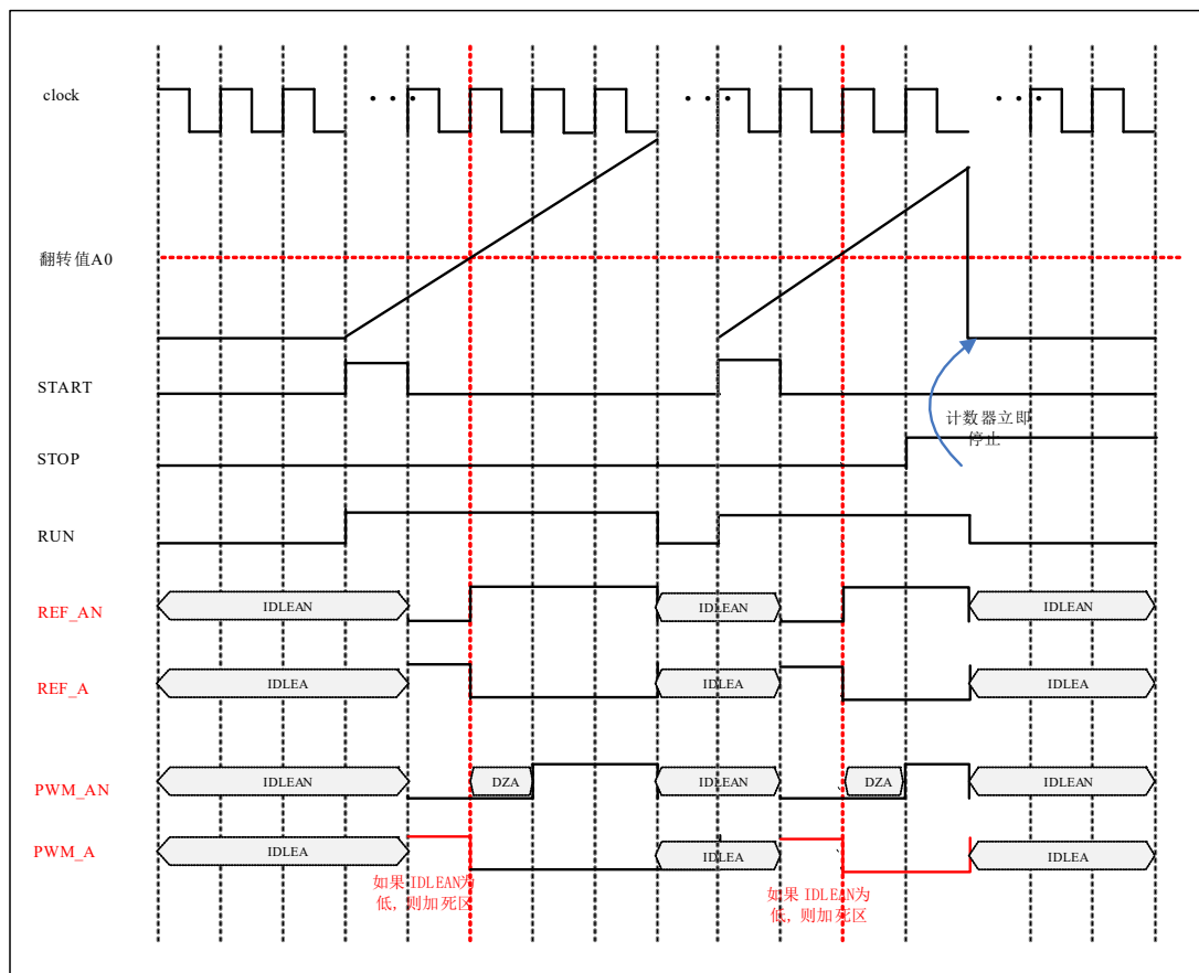
图 6-61 边沿对齐模式下向上计数时计数器启动与停止波形
