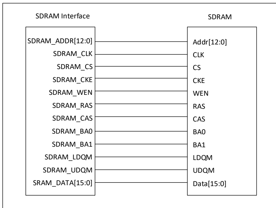
图 6-102 SDRAM 与设备连接示意图
