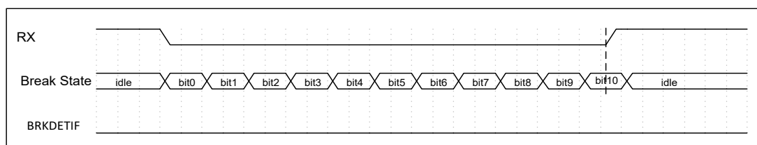
图 6-36 Break 信号不够长示意图
