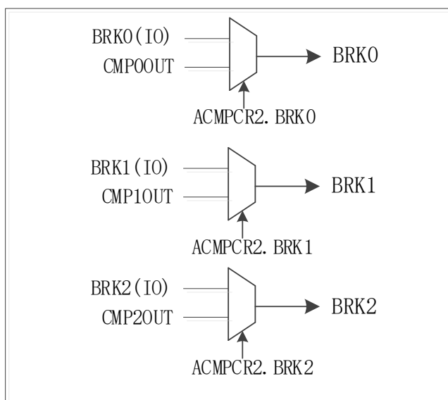
图 6-130 BRK 对应关系图
