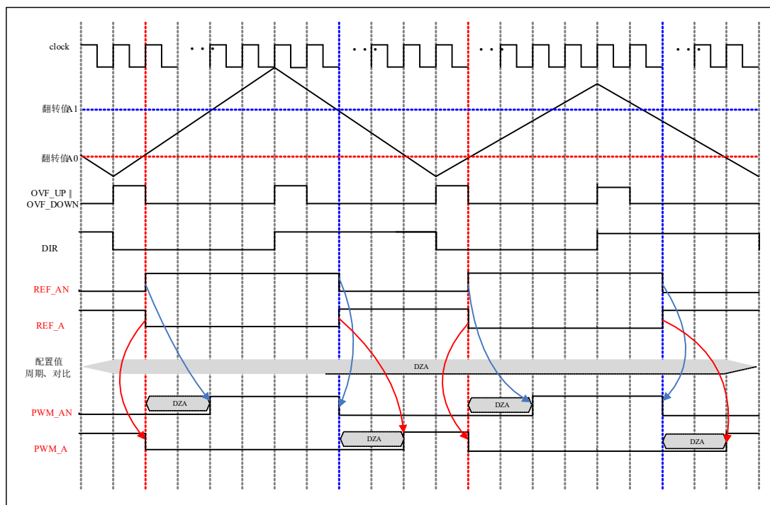
图 6-72 非对称中心对齐模式下 PWM 信号产生波形
