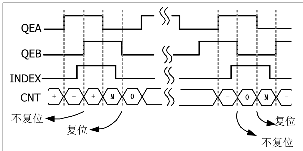
图 6-25 计数匹配复位模式
