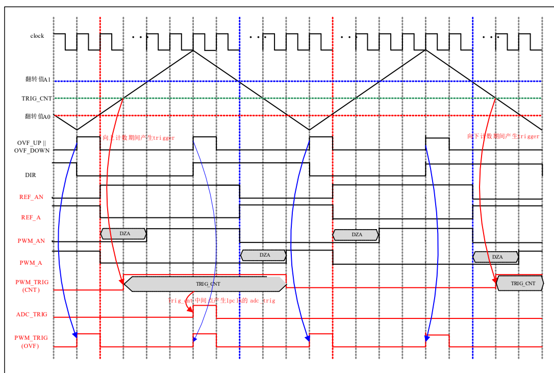
图 6-74 TRIGGER 控制波形
