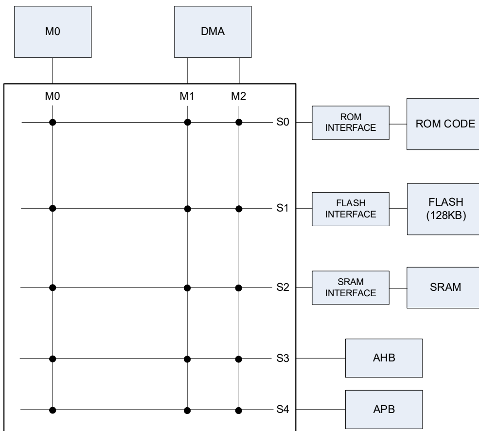
图 4-2 总线矩阵
