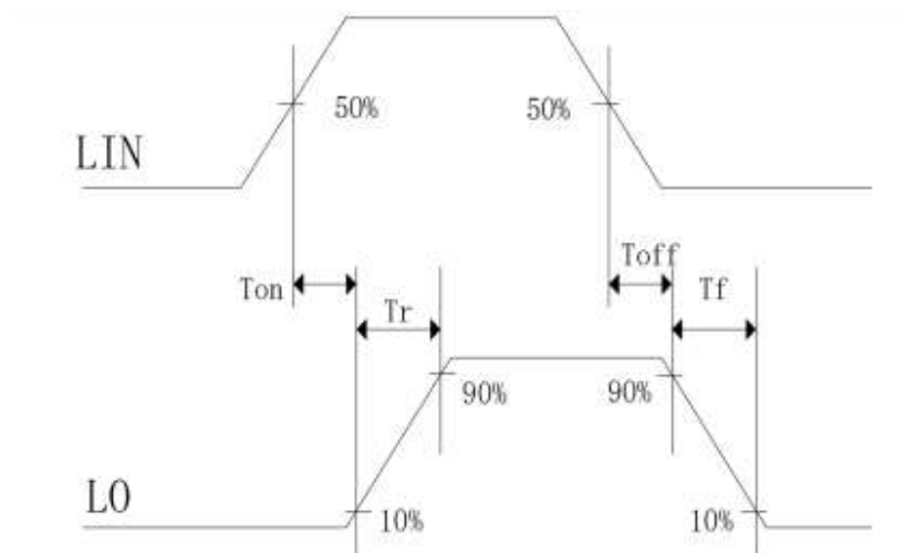
图 10-5 低端输出 LO 开关时间波形图
