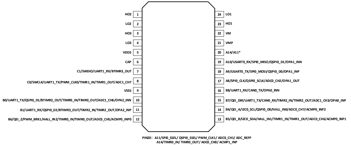
图 5-4 SWM22PE8S7 封装管脚配置图
