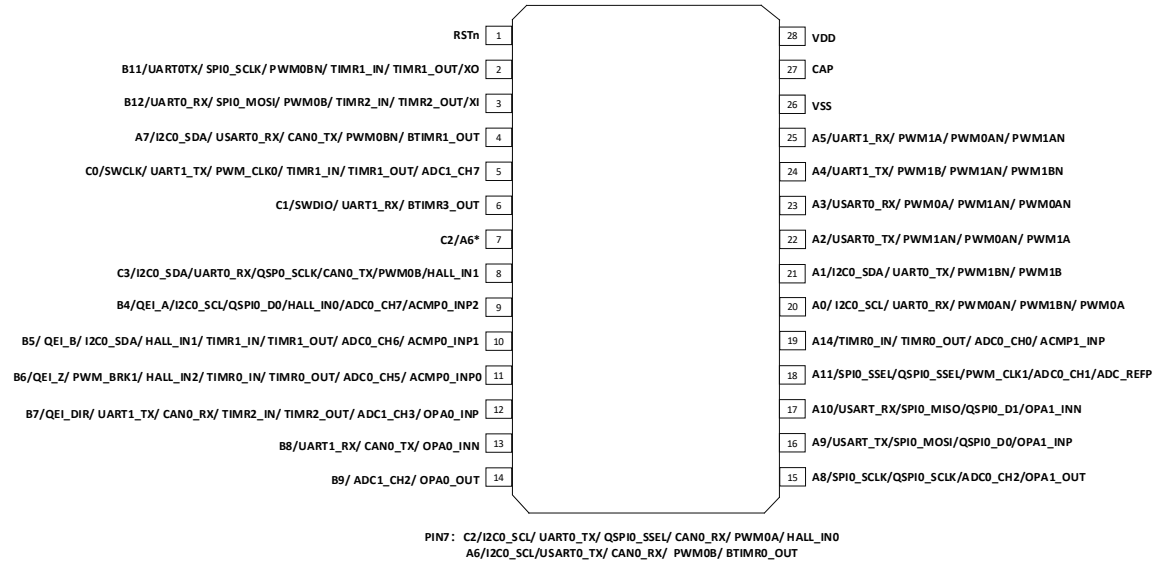
图 5-7 SWM221GBS7 封装管脚配置图 4
