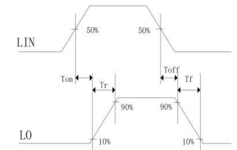
图 10-6 高端输出 HO 开关时间波形图
