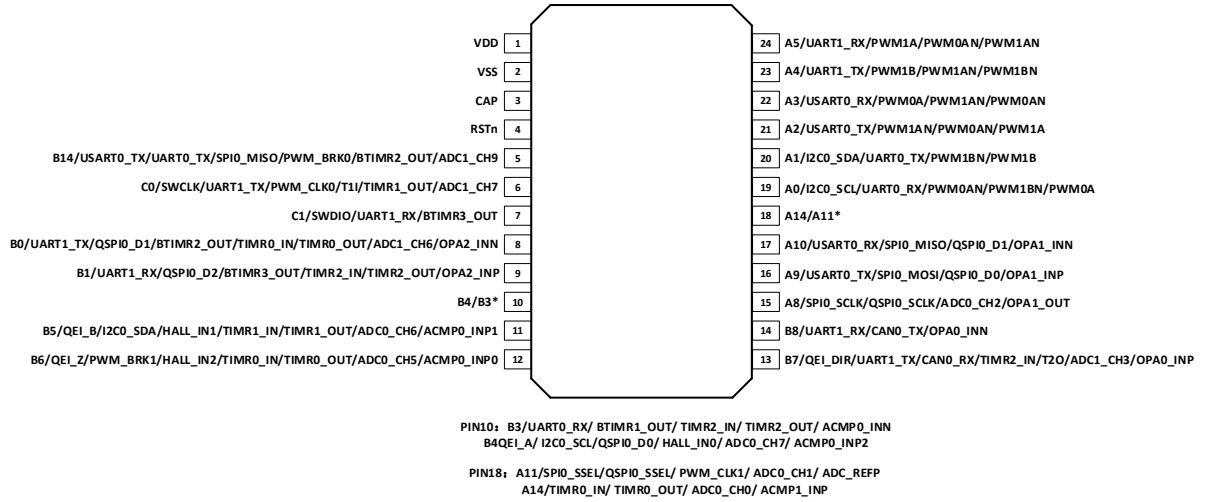
图 5-2 SWM221EBS7 封装管脚配置图
