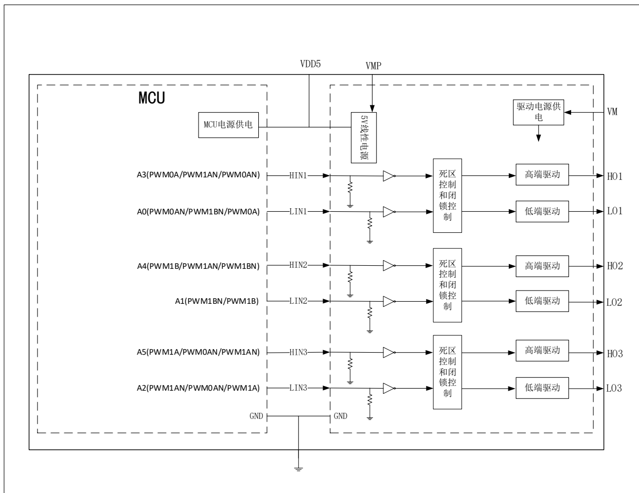
图 7-1 预驱电路结构框图
