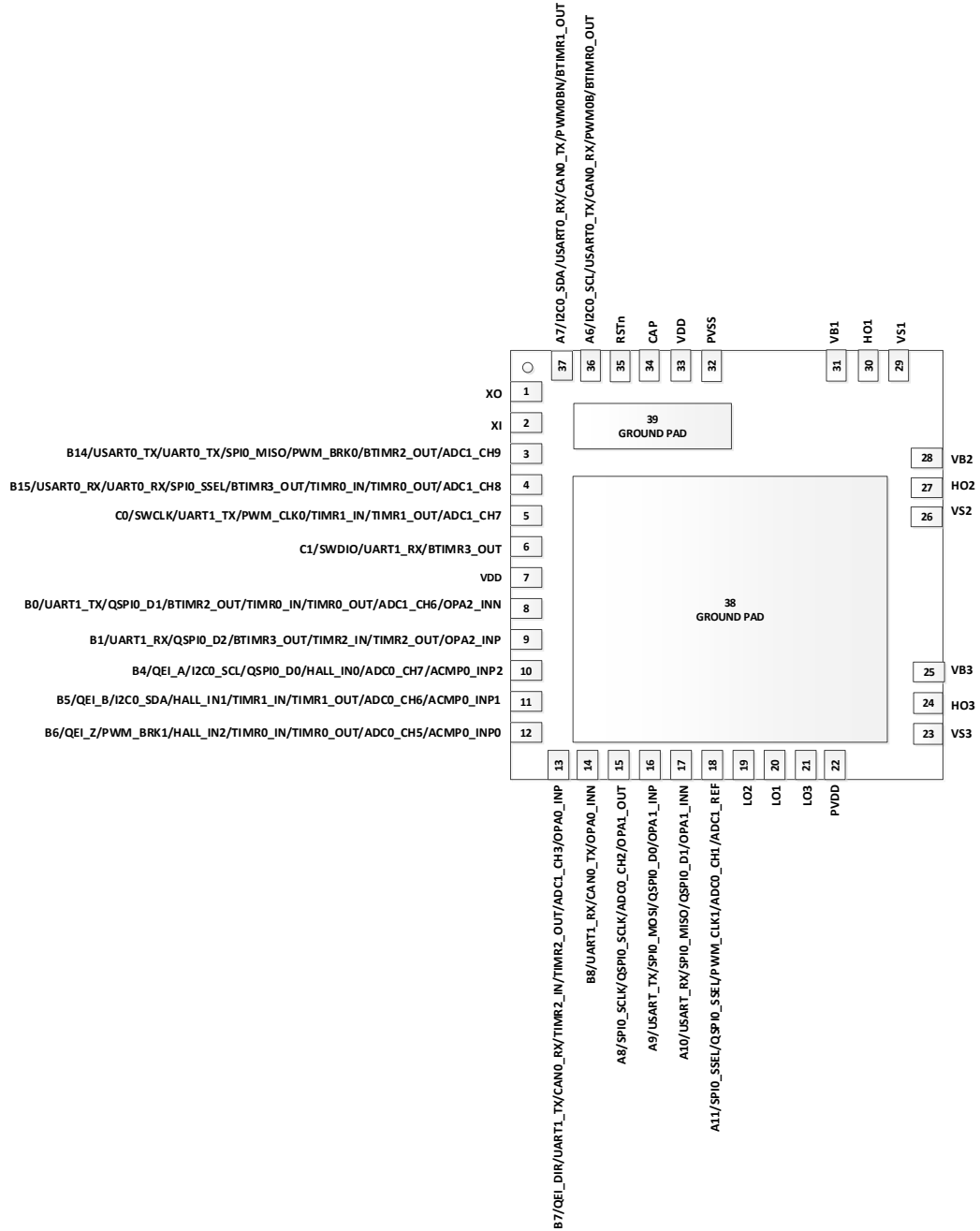
图 5-8 SWM22DC8U7 封装管脚配置图
