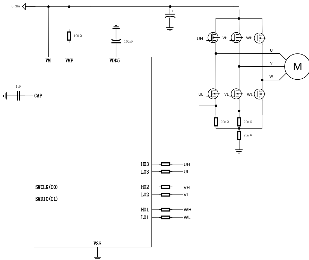
图 7-2 参考应用电路
