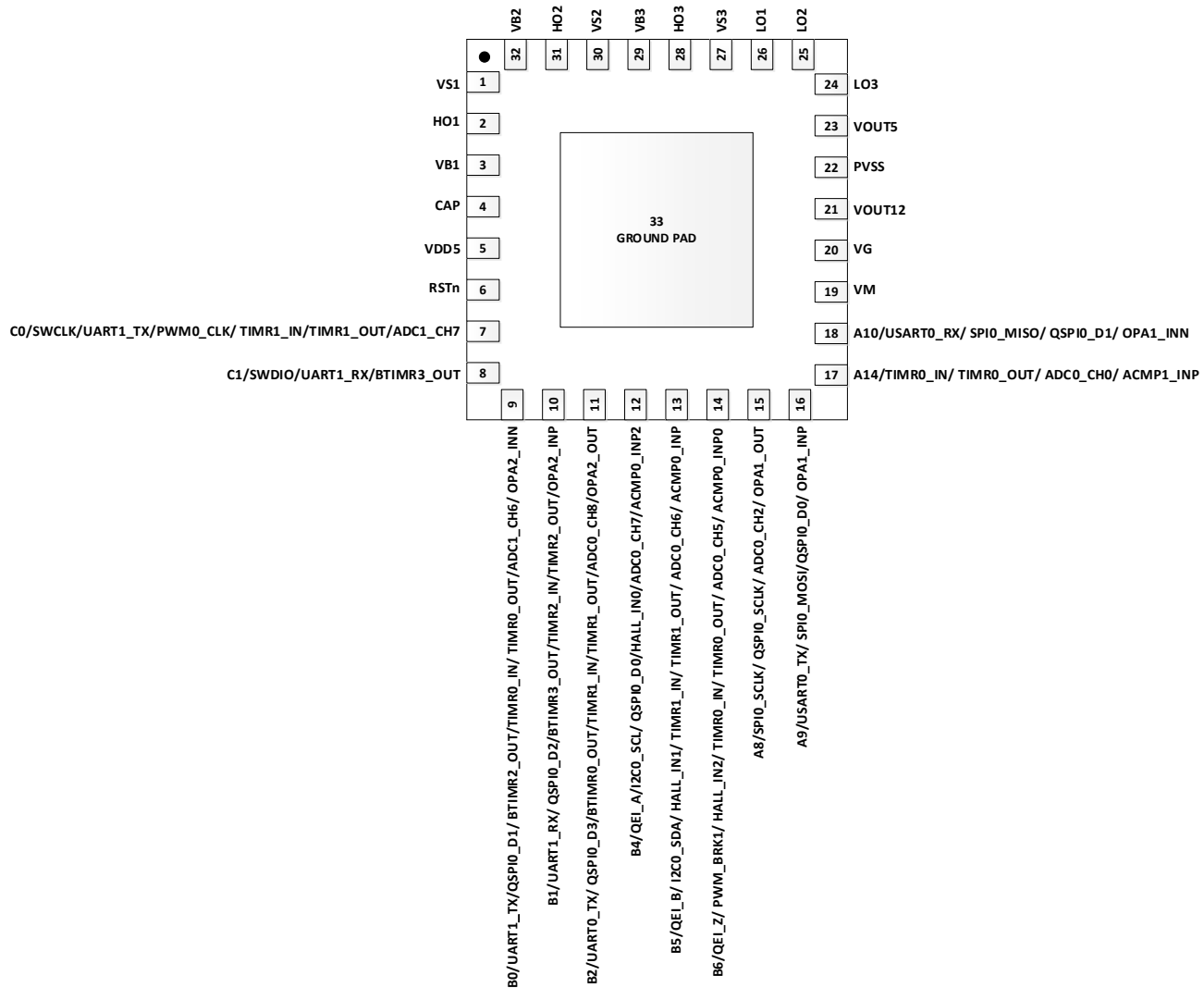
图 5-9 SWM22DK8U7 封装管脚配置图
