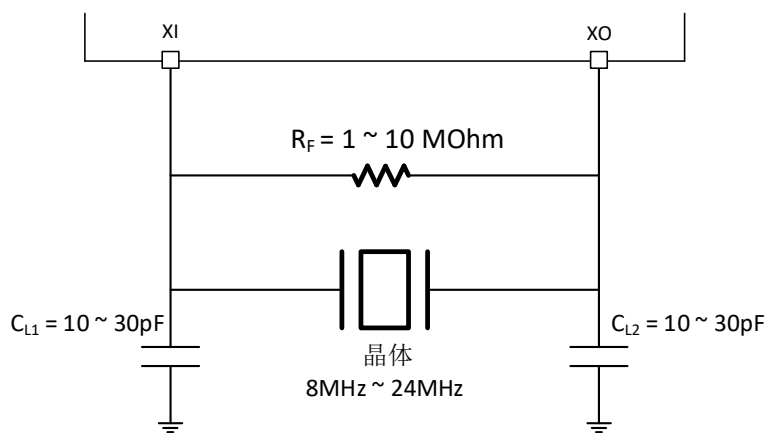
图 10-1 外部晶体振荡器典型电路
