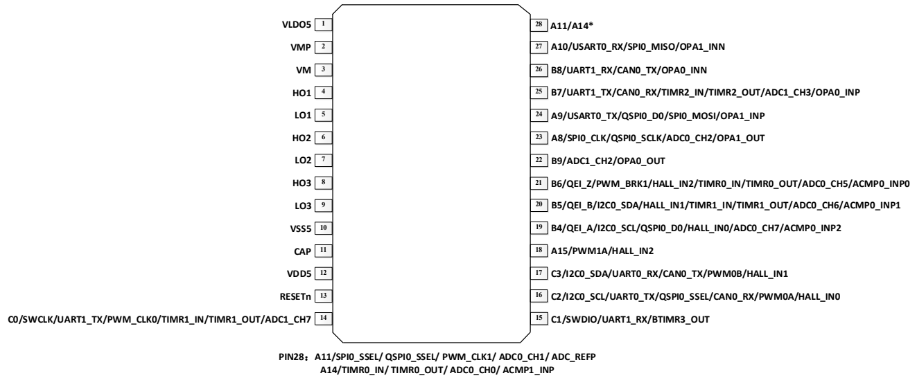
图 5-6 SWM22PG8S7 封装管脚配置图
