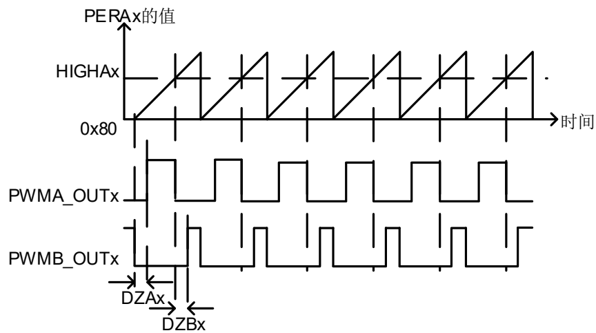
图 6-41 开启死区的互补模式
