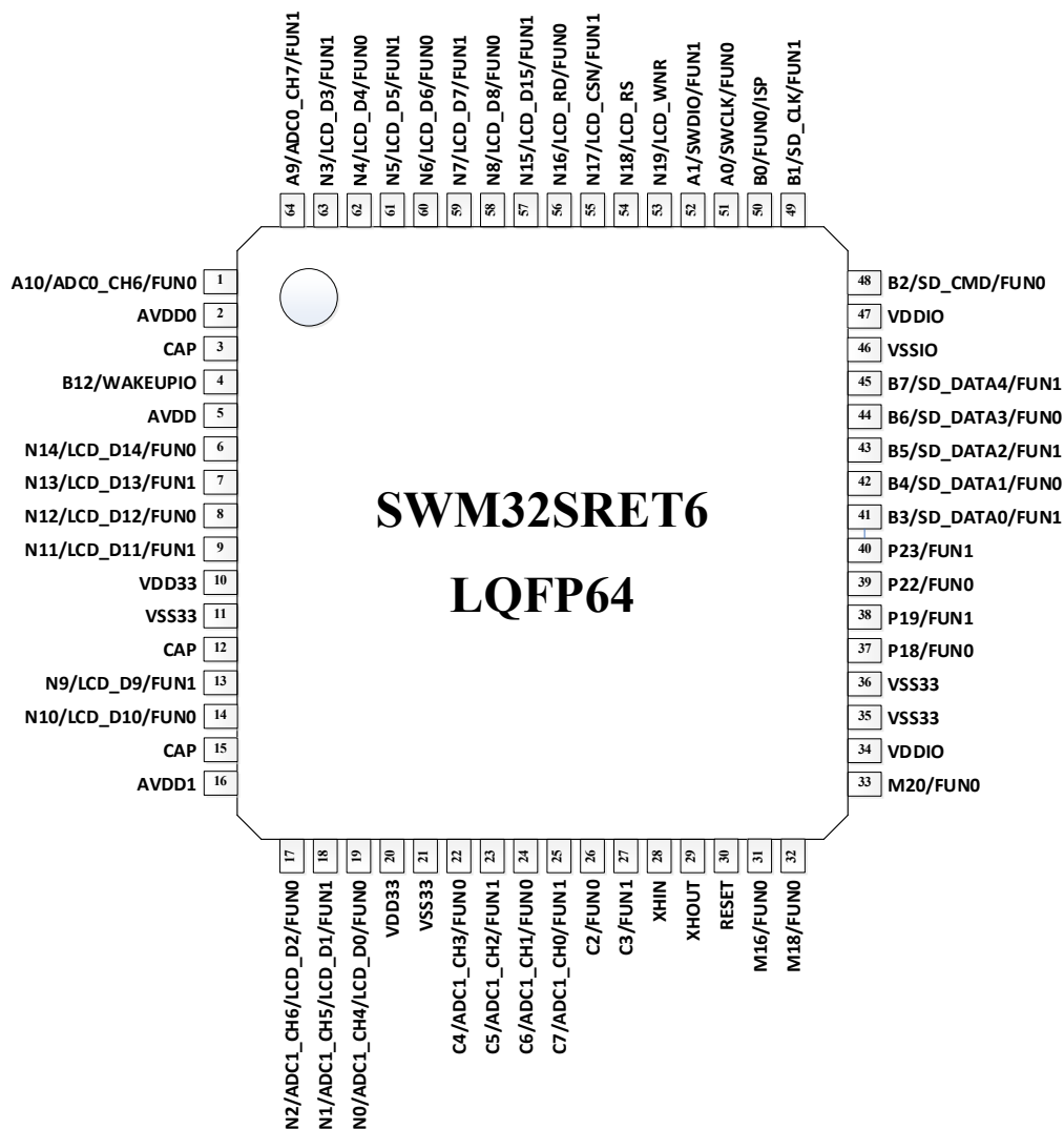
图表 1 SWM32SRET6 1
