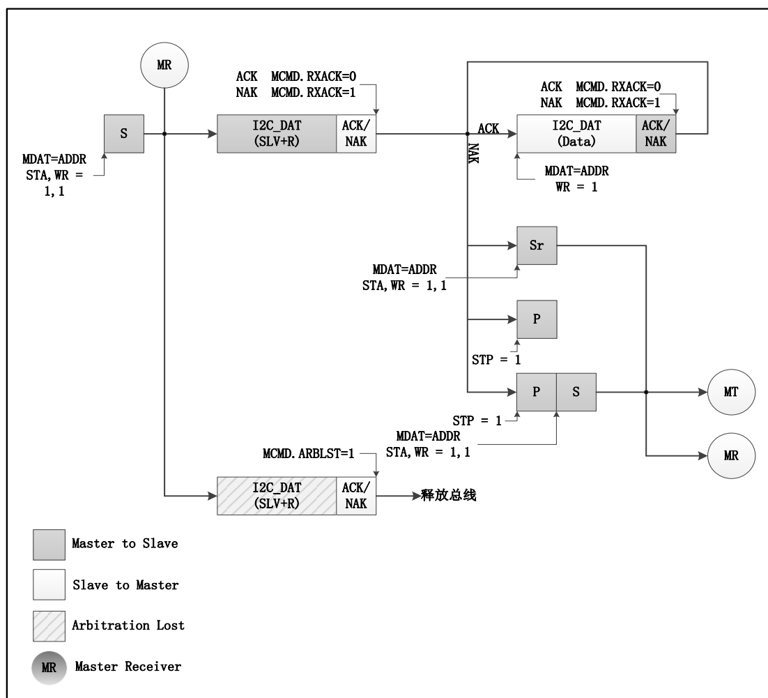
图 6-30 主机接收/从机发送流程
