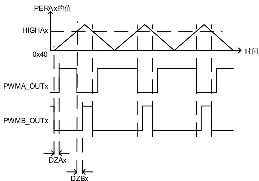
图 6-44 中心对称互补模式
