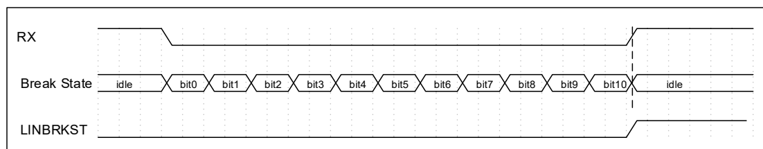
图 6-21 Break 信号恰好够长示意图
