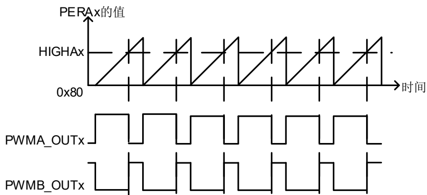
图 6-40 未开启死区的互补模式
