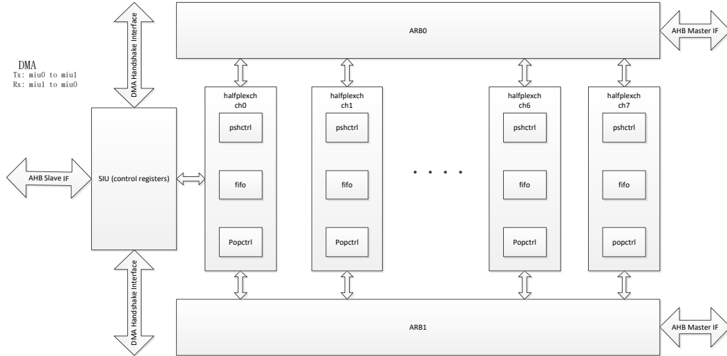
图 6-54 DMA 模块结构图
