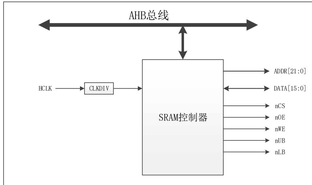
图 6-60 SRAMC 模块结构示意图
