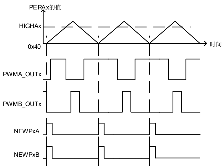
图 6-49 PWM 中心对称互补模式下新周期起始中断示意图
