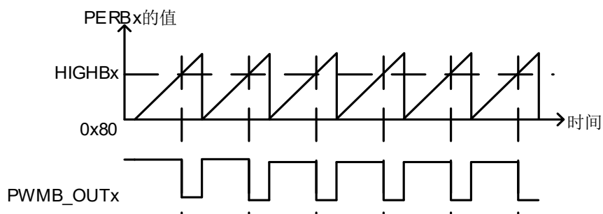
图 6-39 PWM 独立模式起始输出高电平示意图
