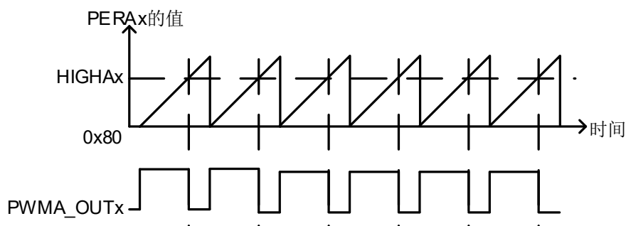
图 6-38 PWM 独立模式起始输出低电平示意图
