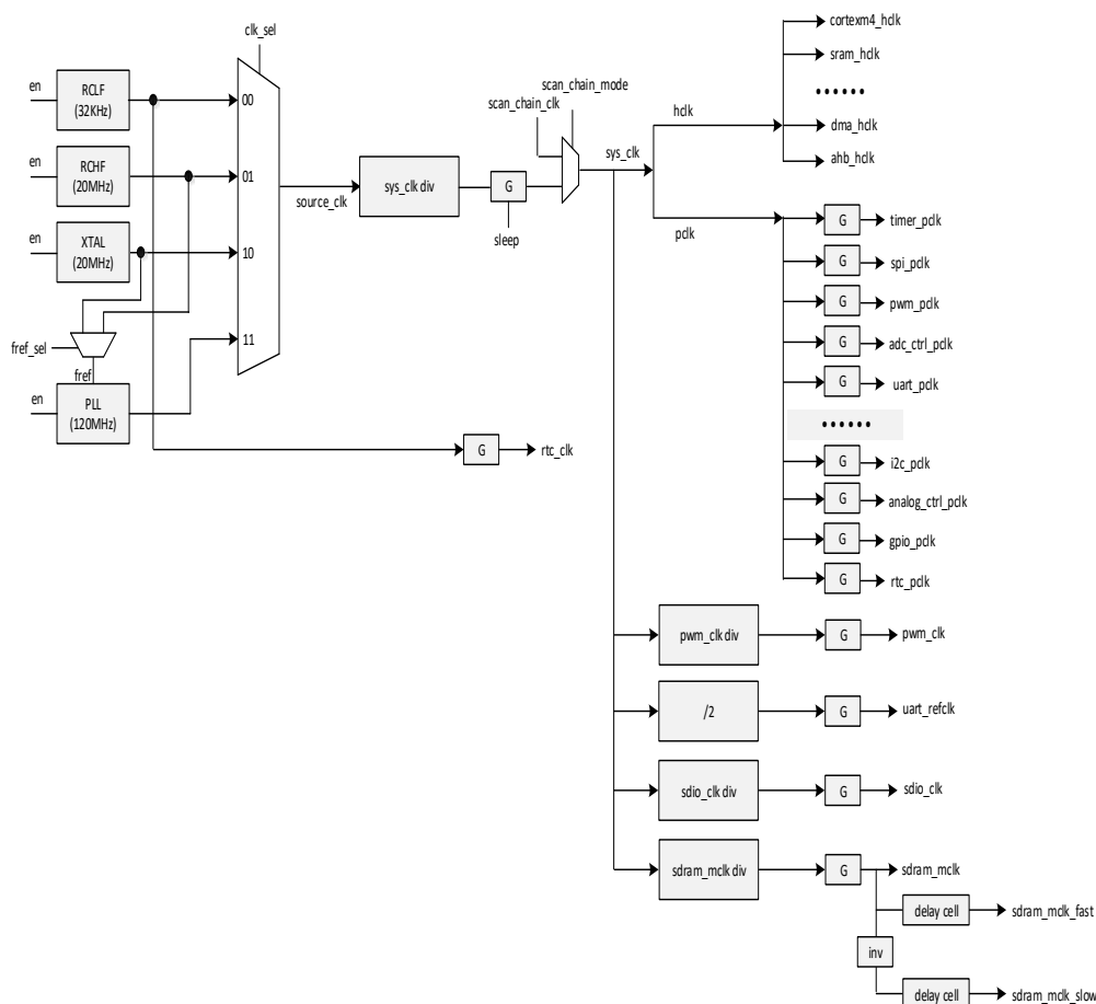
图 6-3 时钟连接图
