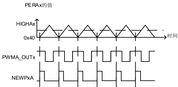
图 6-48 PWM 中心对称模式下新周期起始中断示意图
