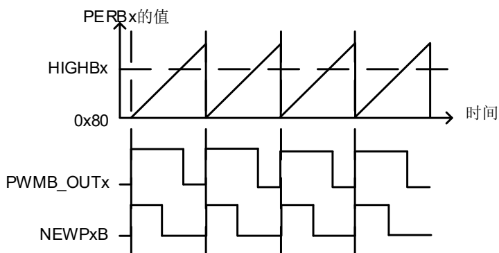
图 6-47 PWM 独立模式下新周期起始中断示意图
