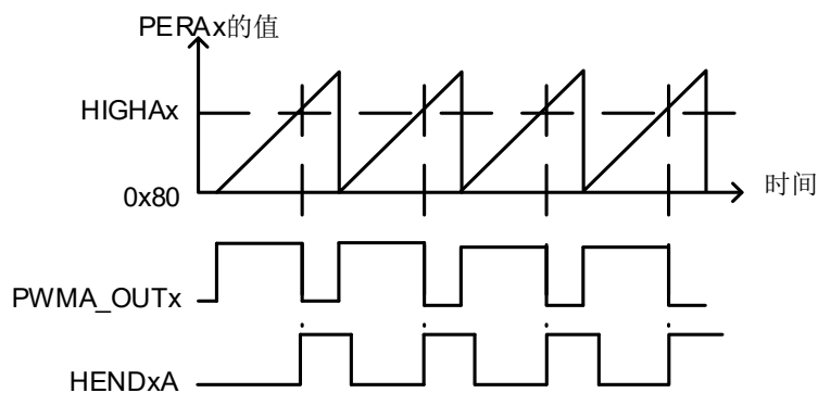
图 6-46 PWM 独立模式下高电平结束中断示意图
