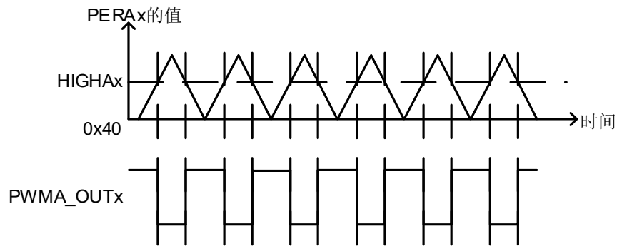
图 6-42 中心对称模式
