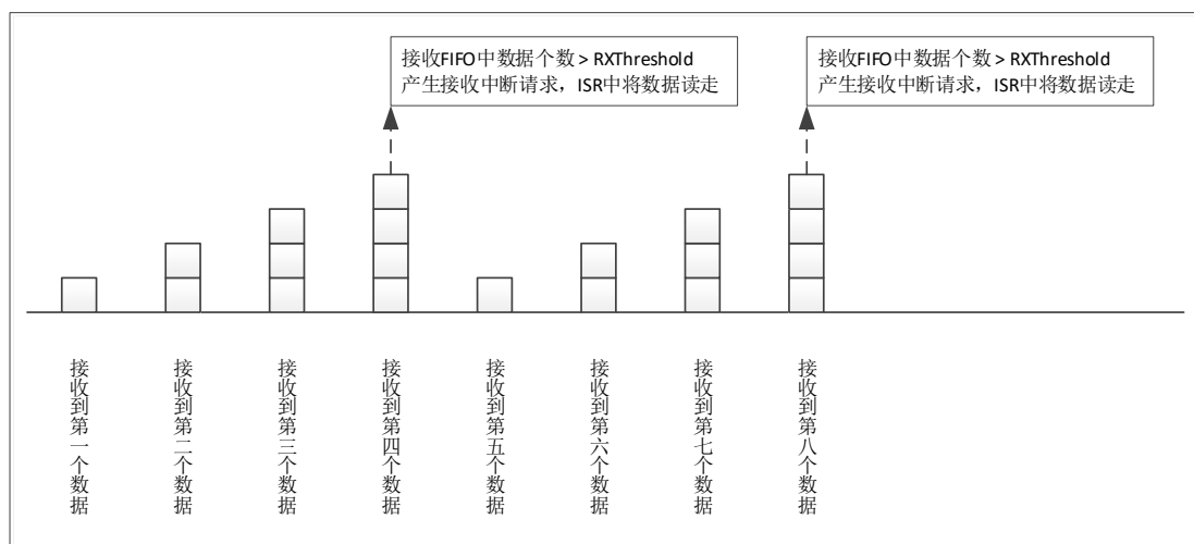
图 6-24 对方发送 8 个数据接收 FIFO 示意图
