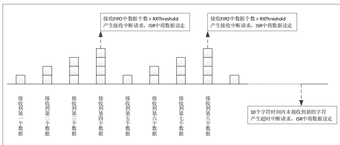
图 6-25 对方发送 9 个数据接收 FIFO 示意图
