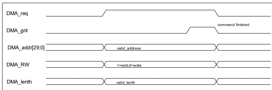
图 6-55 DMA 访问外设握手时序示意图
