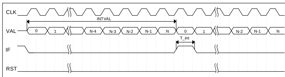
图 6-25 WDT 配置为中断模式波形图
