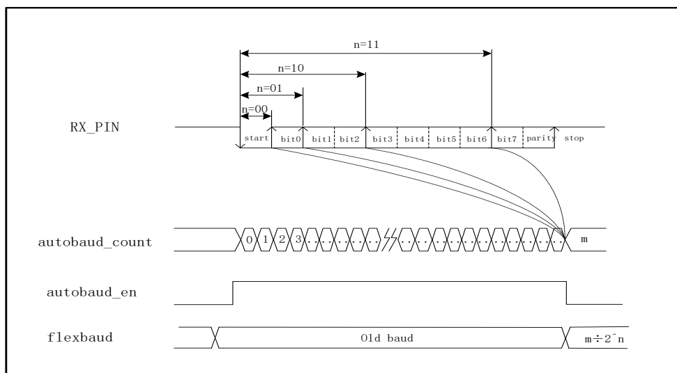
图 6-29 自动波特率示意图
