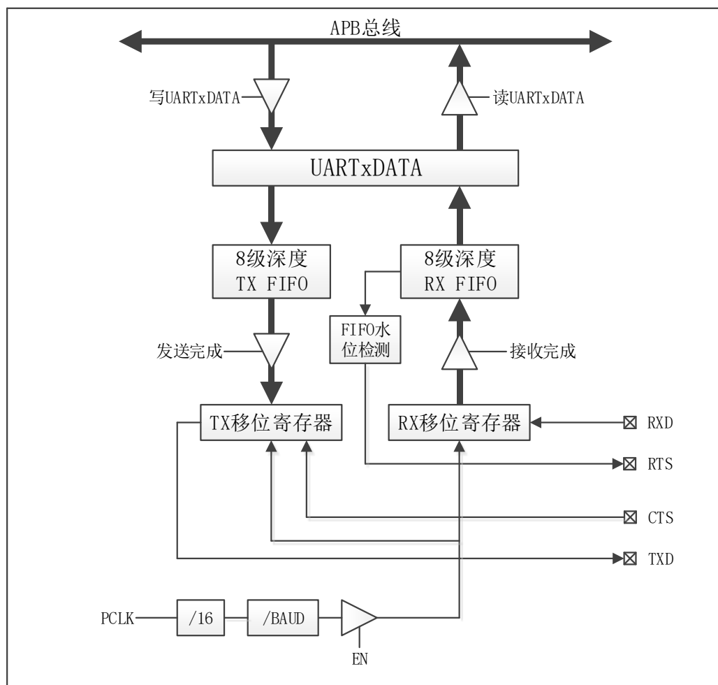
图 6-27 UART 模块结构图
