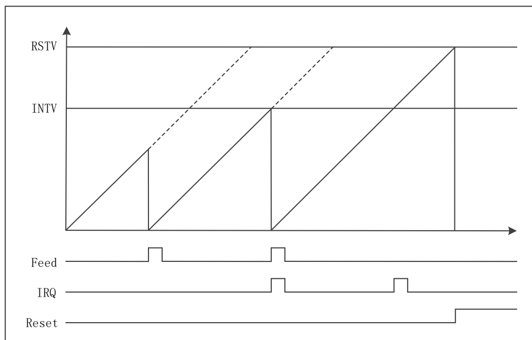
图 6-23 WDT 工作示意图
