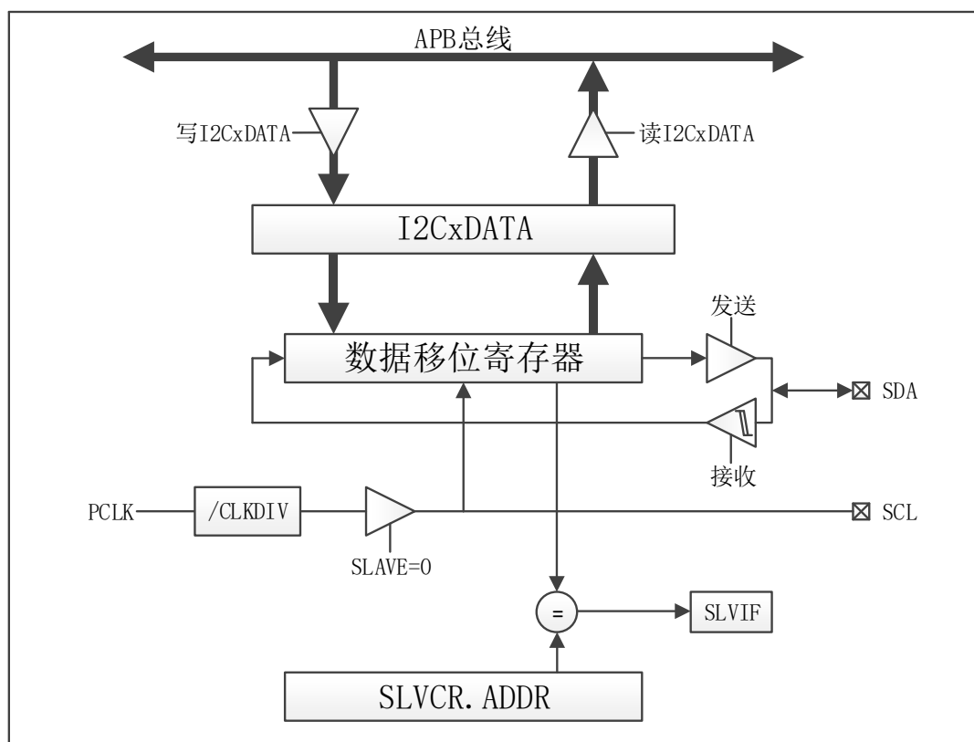
图 6-38 I2C 模块结构框图
