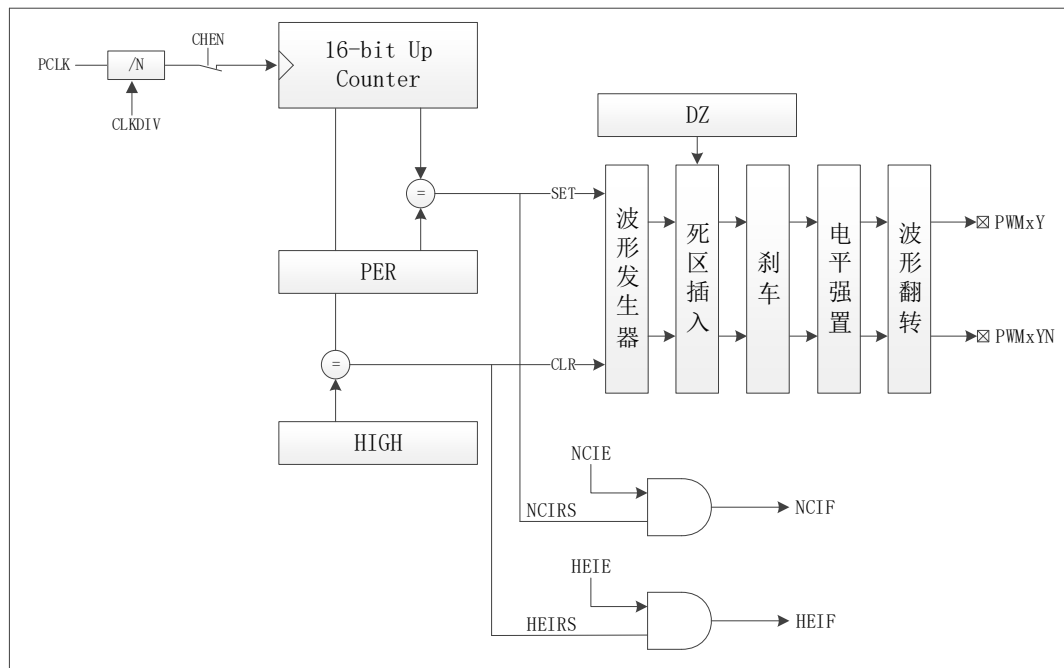
图 6-46 PWM 模块结构框图
