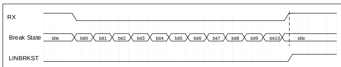
图 6-33 Break 信号足够长示意图
