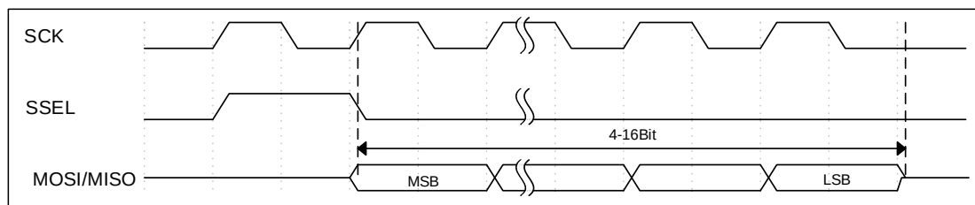
图 6-44 SSI 模式单次输出波
