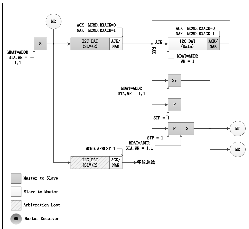
图 6-41 主机接收/从机发送流程
