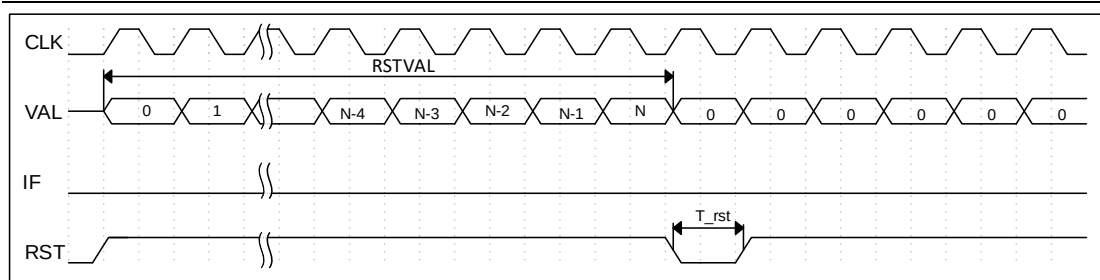
图 6-24 WDT 配置为 RESET 模式波形图
