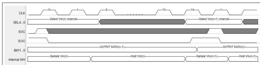
图 6-59 SAR ADC 连续采样示意图
