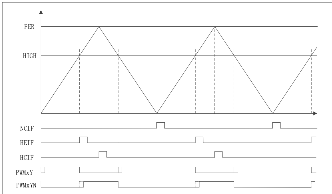
图 6-49 中心对称模式带死区
