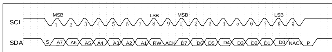
图 6-39 I2C 通信示意图
