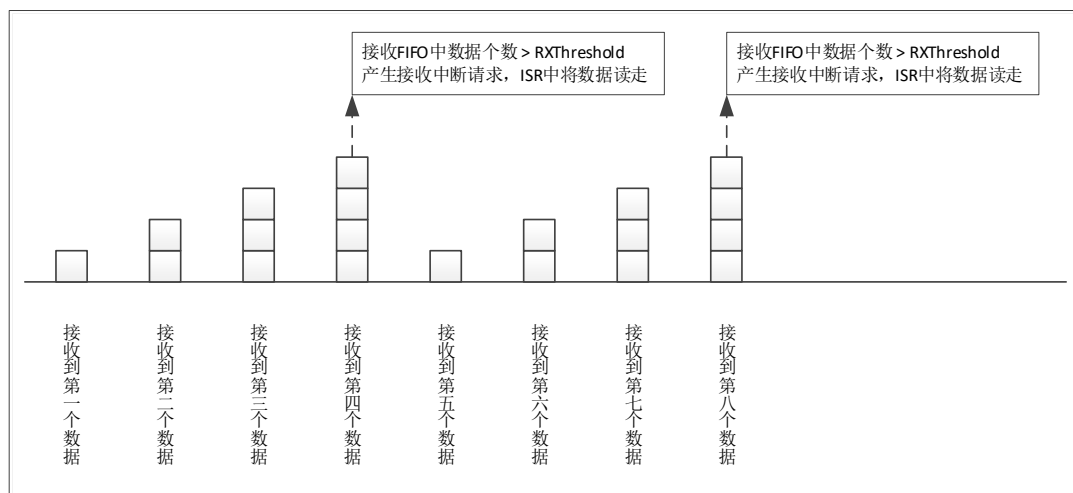
图 6-35 对方发送 8 个数据接收 FIFO 示意图
