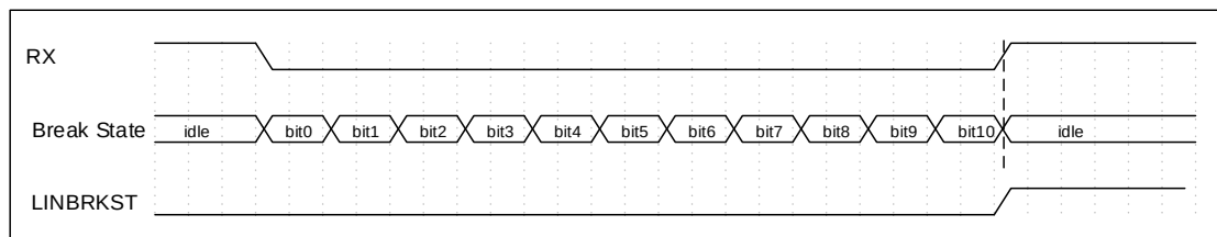
图 6-32 Break 信号恰好够长示意图
