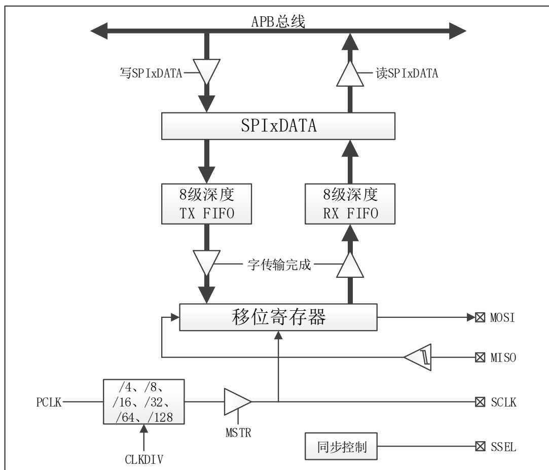
图 6-42 SPI 模块结构框图
