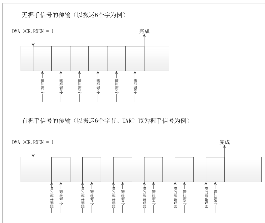
图 6-63 握手、非握手信号传输图
