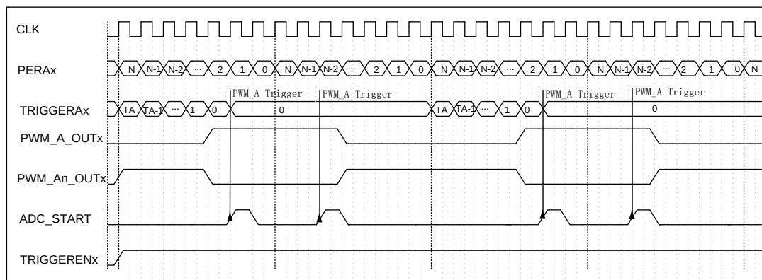
图 6-52 PWM 触发 ADC 采样示意图
