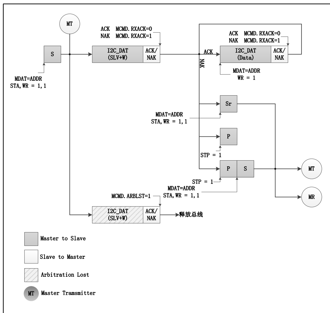
图 6-40 主机发送/从机接收流程
