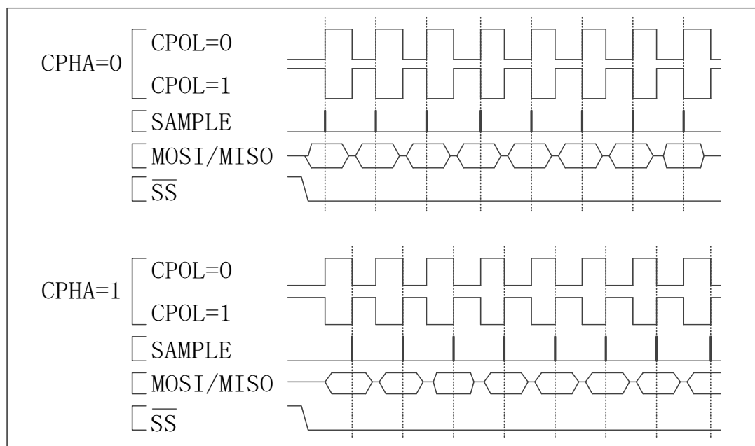
图 6-43 SPI 模式波形图
