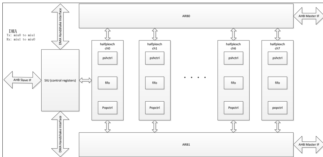
图 6-61 DMA 模块结构图
