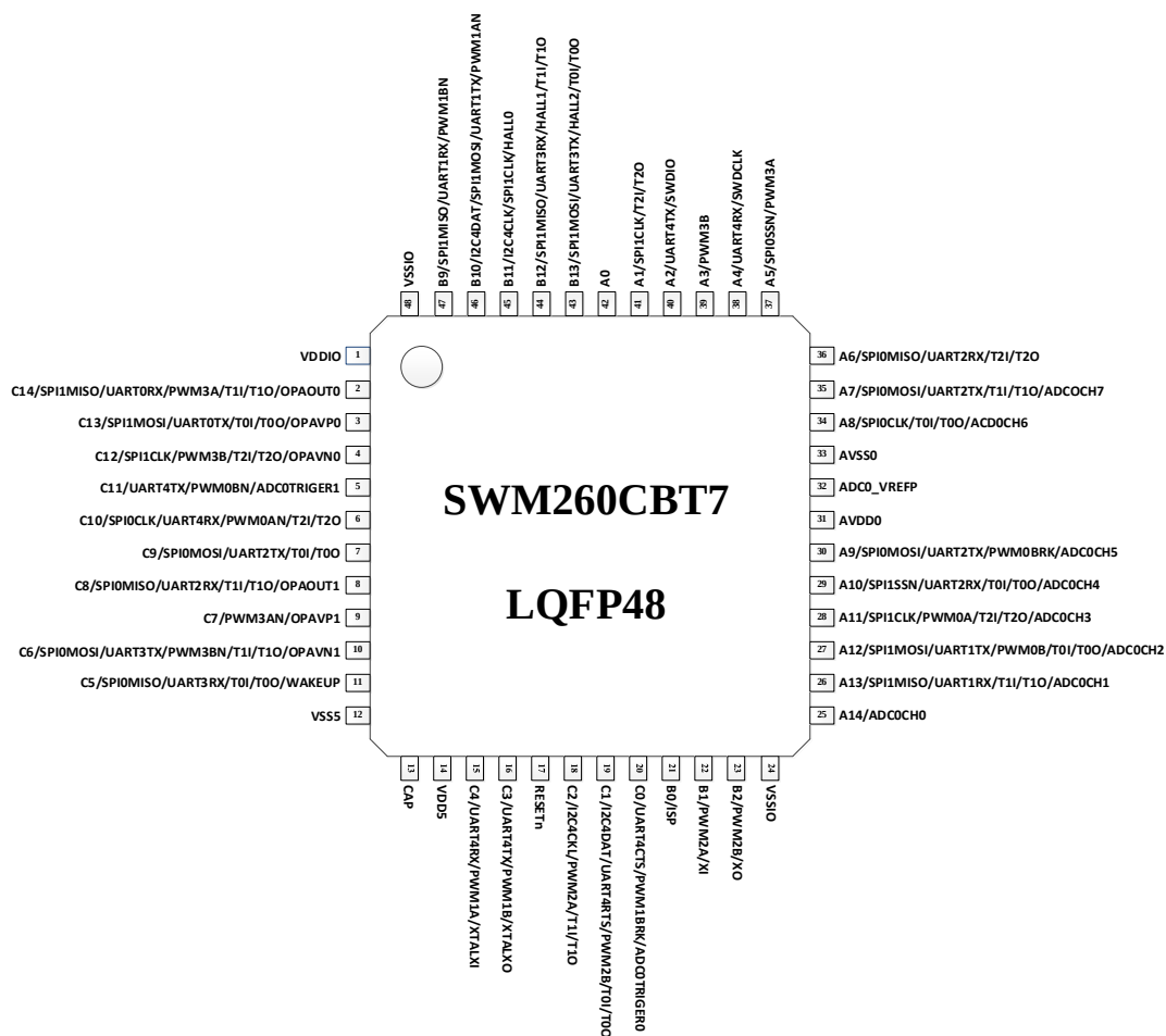
图 5-1 CBT7 封装管脚配置图
