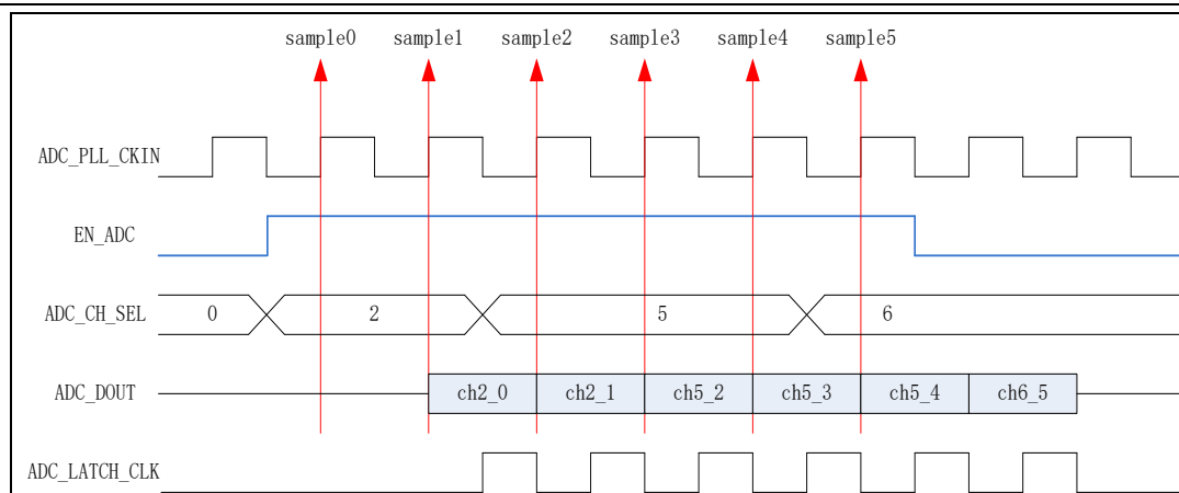
图 6-60 SAR ADC 多通道连续采样示意图
