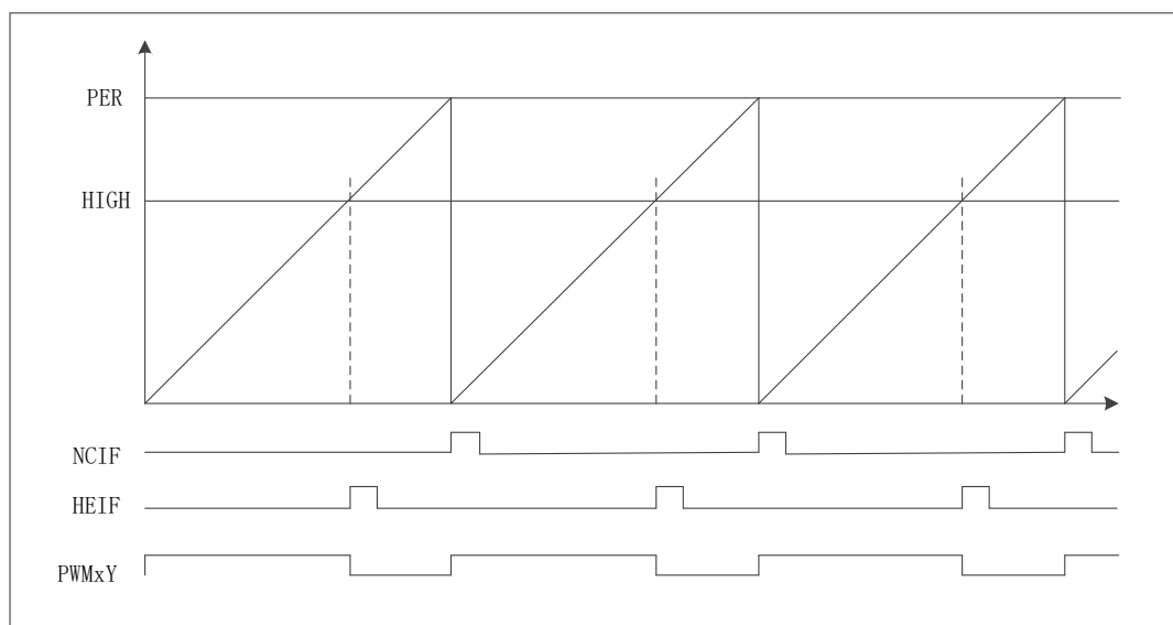
图 6-48 边沿模式
