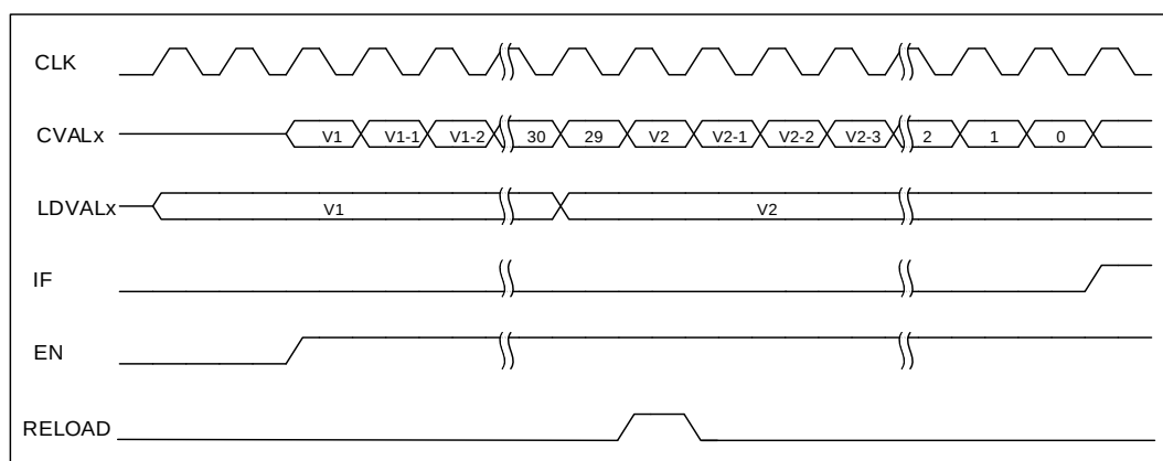
图 6-21 定时器 RELOAD 工作示意图
