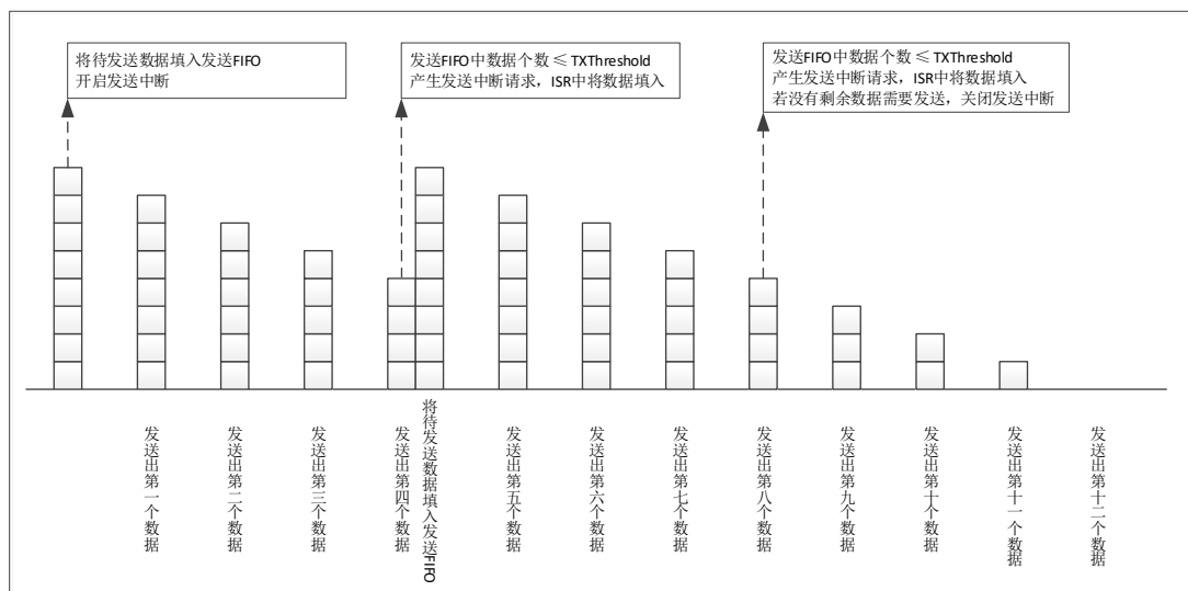
图 6-37 发送 FIFO 示意图
