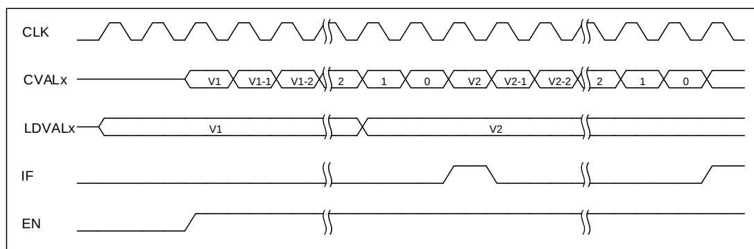
图 6-20 定时器工作示意图
