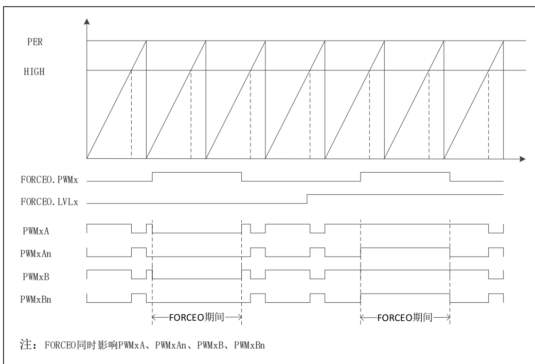
图 6-53 输出屏蔽功能示意图
