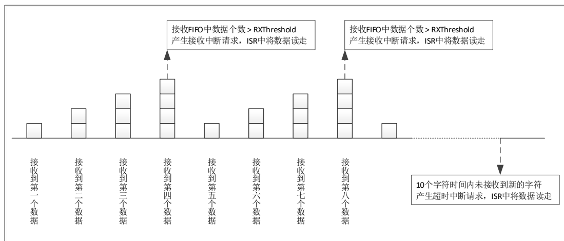
图 6-36 对方发送 9 个数据接收 FIFO 示意图
