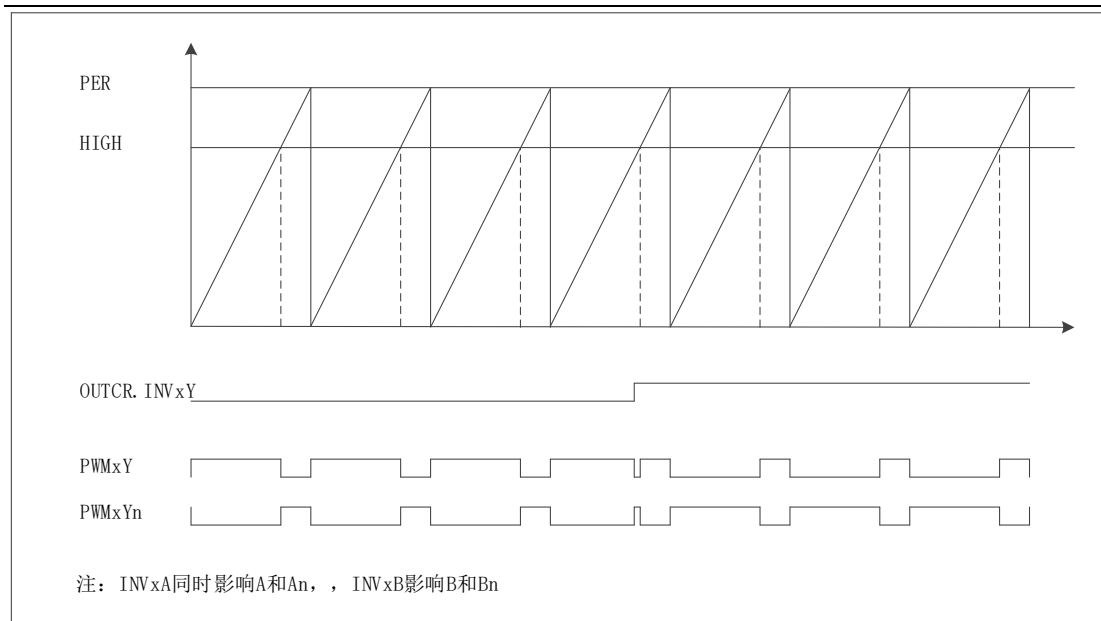
图 6-56 电平翻转示意图
