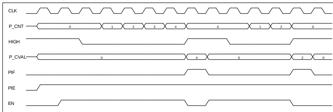
图 6-17 单次低电平捕捉示意图
