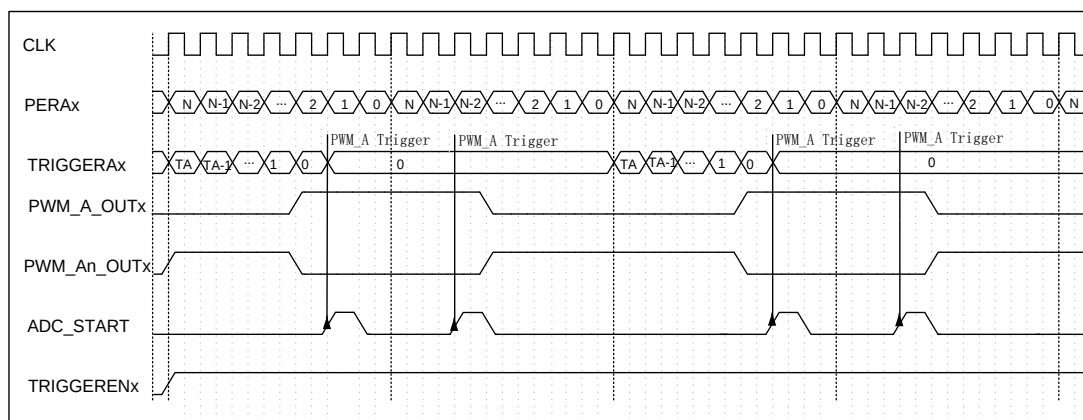
图 6-58 中心对称模式下 PWM 触发 ADC 采样示意图
