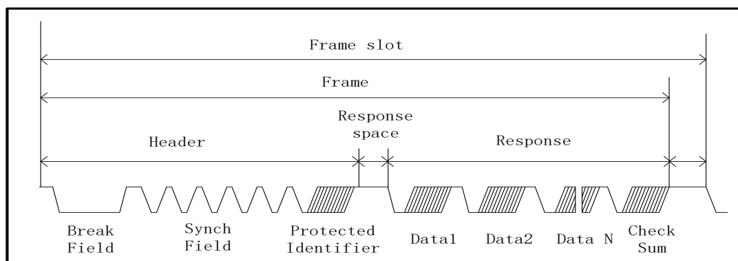
图 6-30 LIN Fram 示意图
