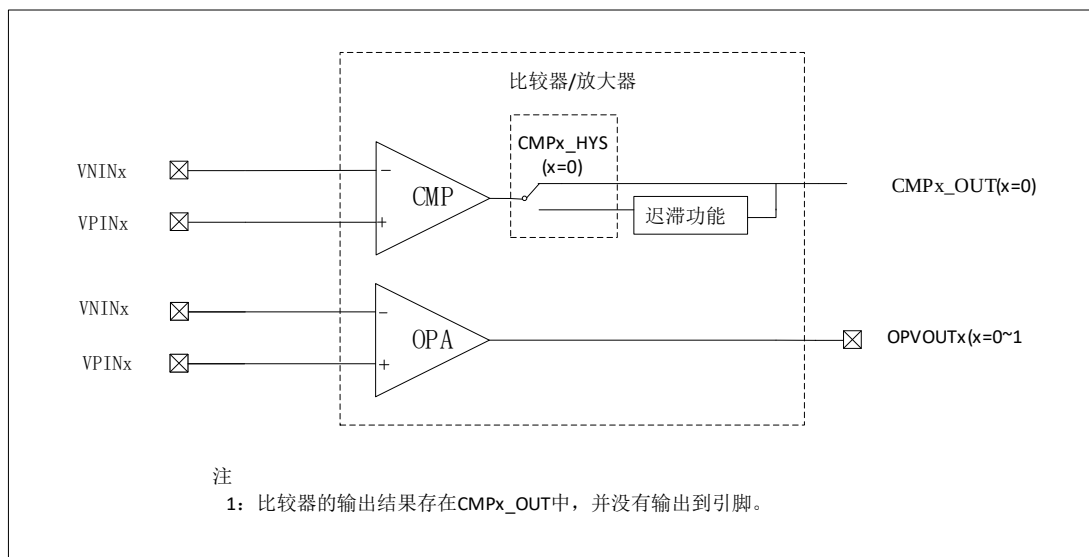
图 6-65 比较器/放大器框图
