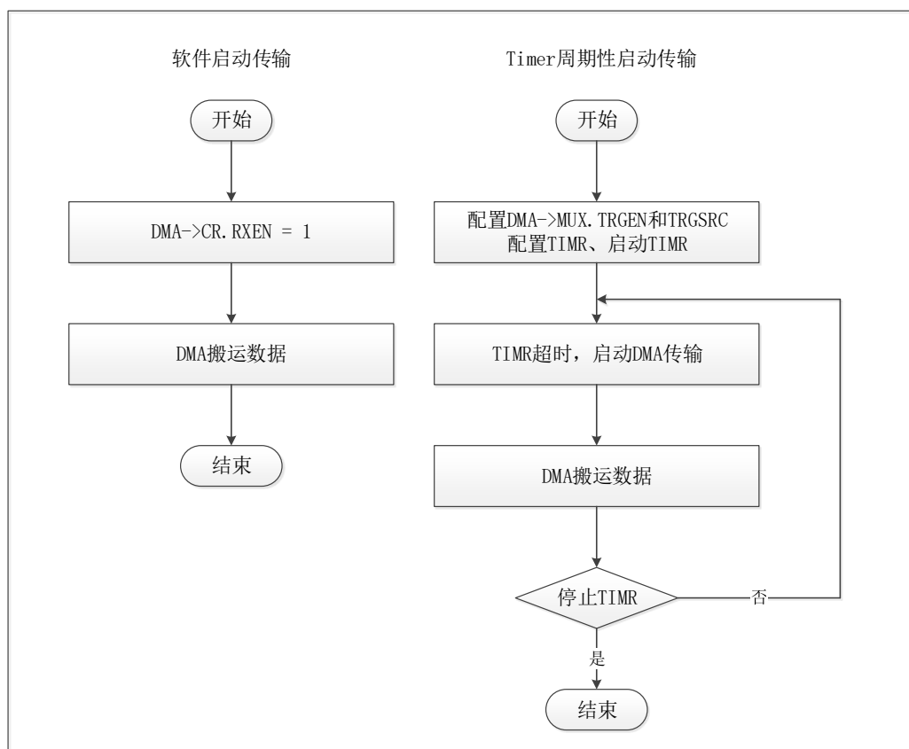
图 6-64 DMA 启动方式
