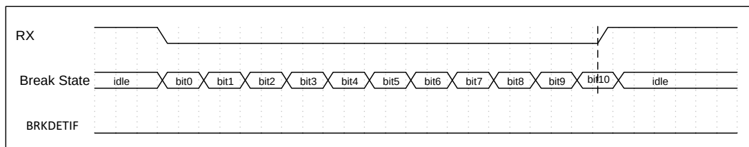
图 6-31 Break 信号不够长示意图
