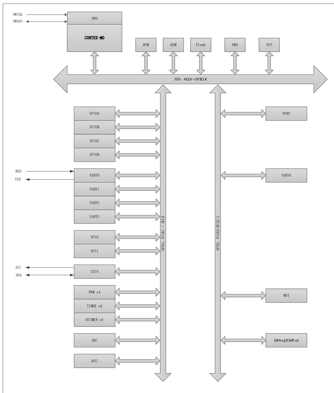
图 4-1 功能方框图
