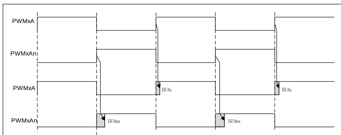
图 6-47 PWM 死区示意图
