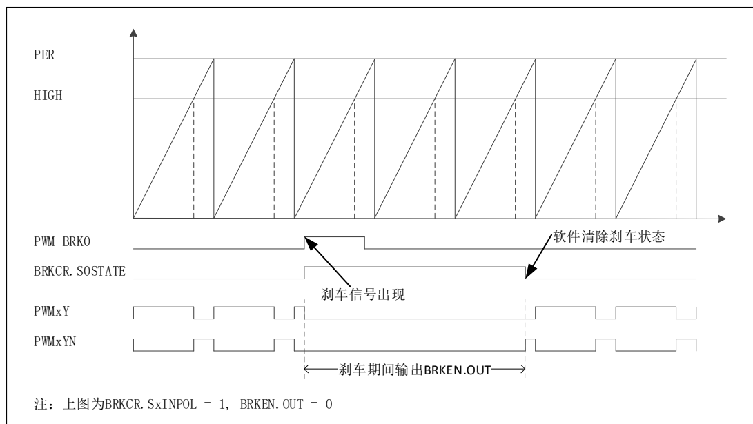
图 6-55 刹车示意图
