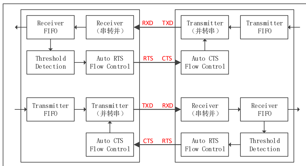
图 6-34 硬件流控
