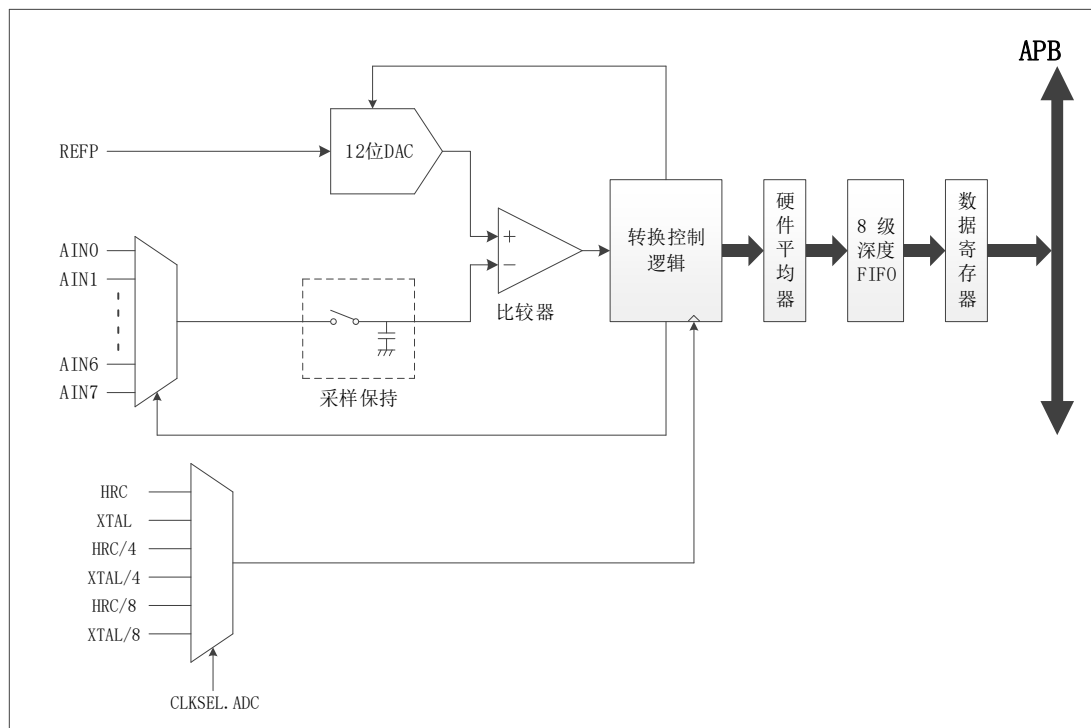
图 6-57 ADC 模块结构框图
