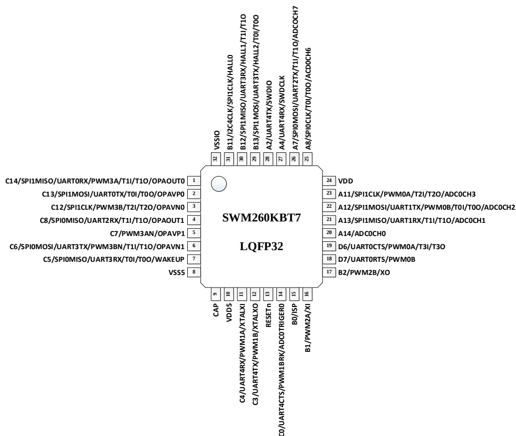
图 5-3 KBT7 封装管脚配置图
