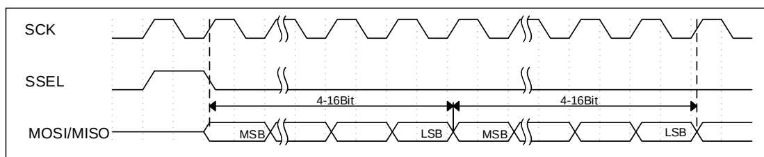
图 6-45 SSI 模式连续输出波形
