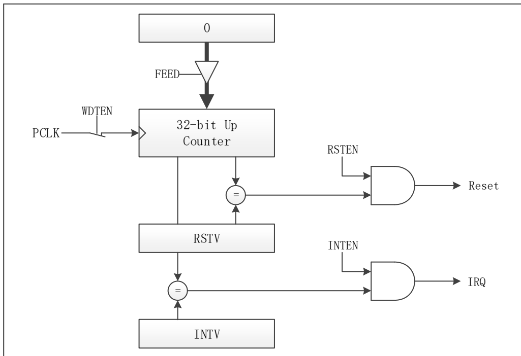
图 6-22 WDT 模块结构框图
