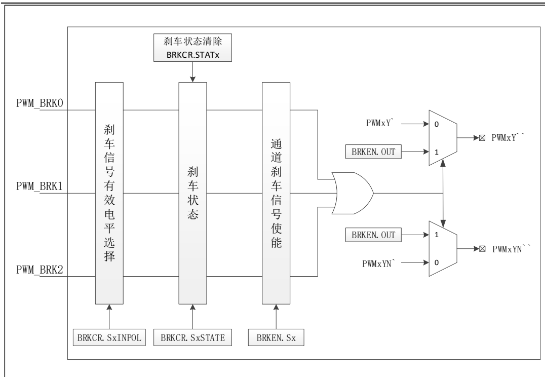
图 6-54 刹车结构图
