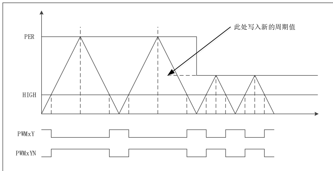
图 6-50 中心对称模式周期结束更新示意图
