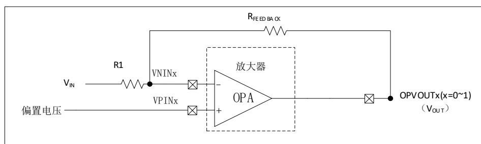
图 6-66 典型放大电路
