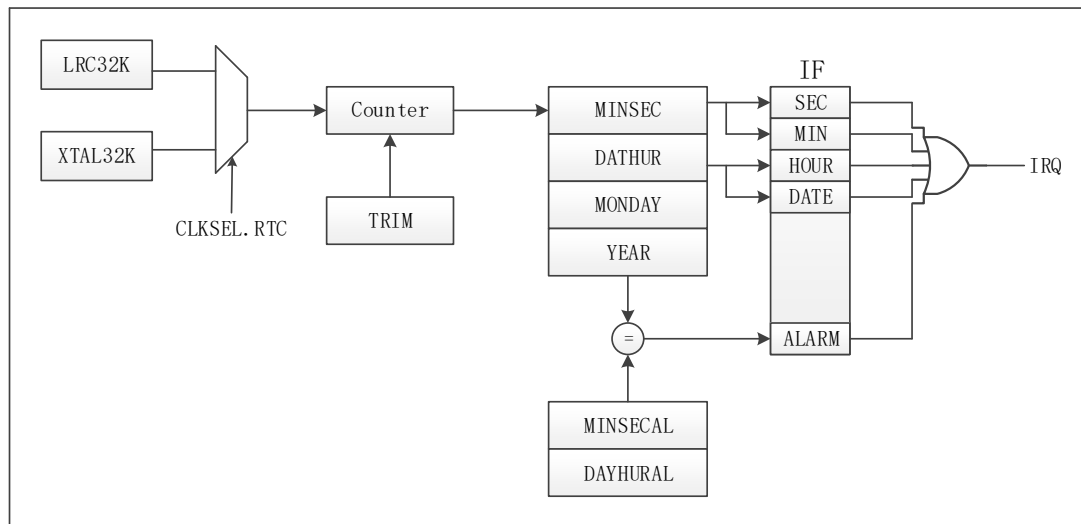
图 6-26 RTC 模块结构框图
