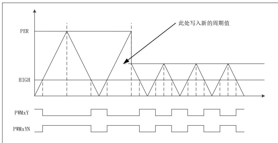
图 6-51 中心对称模式半周期更新示意图
